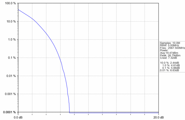
Band7 5MHz QPSK HCH 2567.5MHz RB 25 0 NTN
