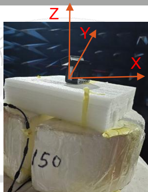
@1575.42MHz
