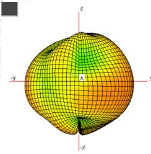
@5850MHz
