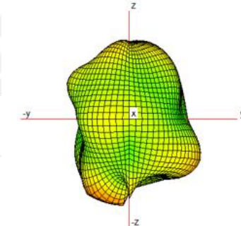
@5850MHz
