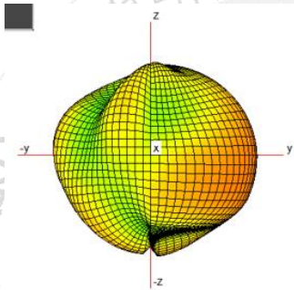
@5450MHz
