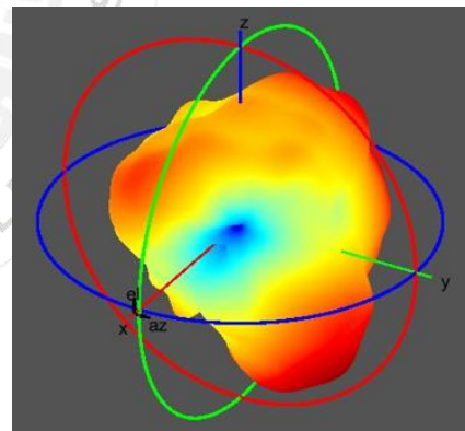
@1602MHz
