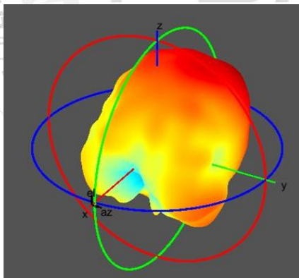
@1575.42MHz
