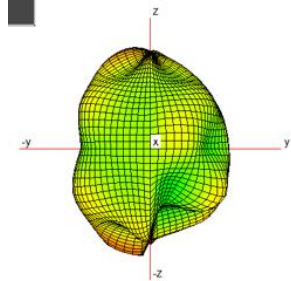
@5150MHz
