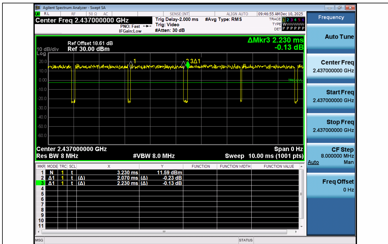
NTNV-11G-Ant1-2437
