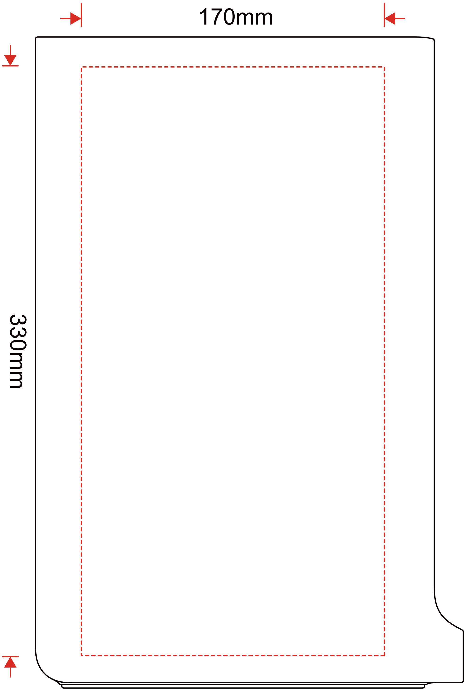
左视图
