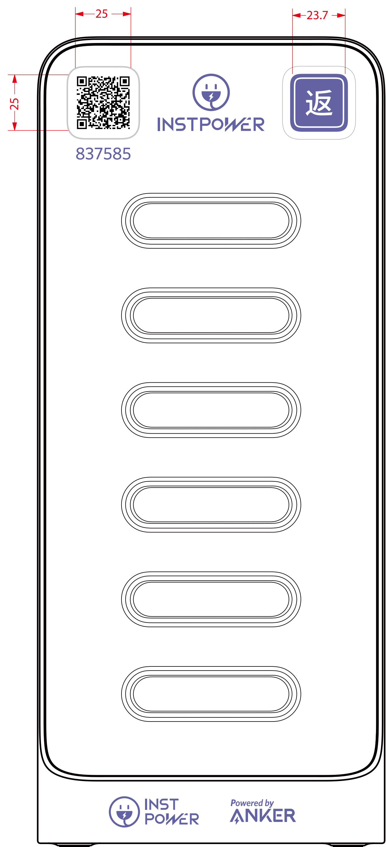
前视图
