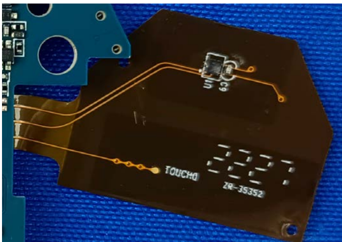
(New NFC module)
