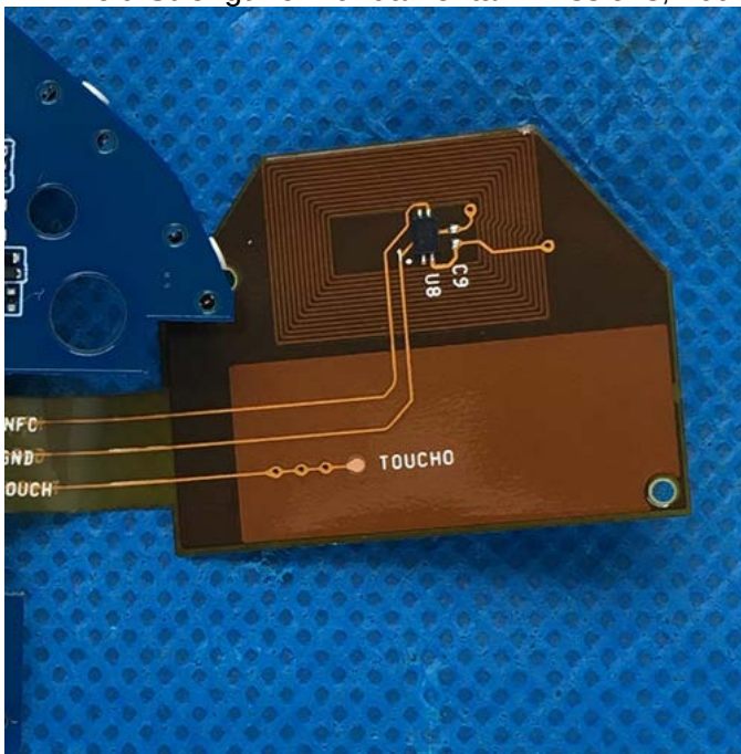
(Old NFC module)
