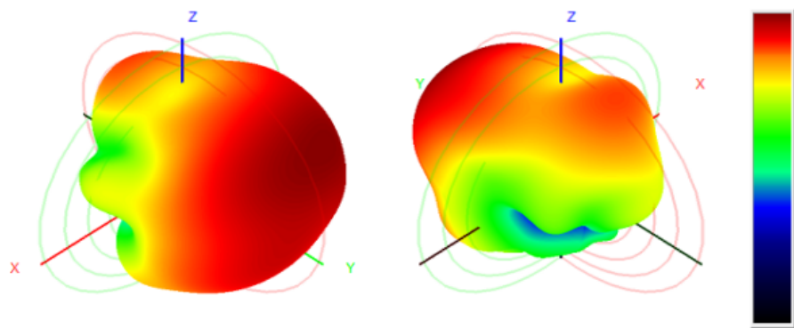
图 3 无源效率方向图 Passive efficiency pattern
