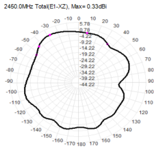
图 4 E1 面-总的增益方向图 E1 plane - total gain pattern
