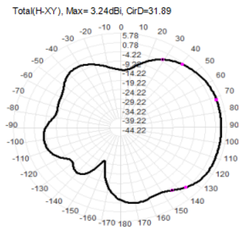
图 6 H 面-总的增益方向图 H plane - total gain pattern
