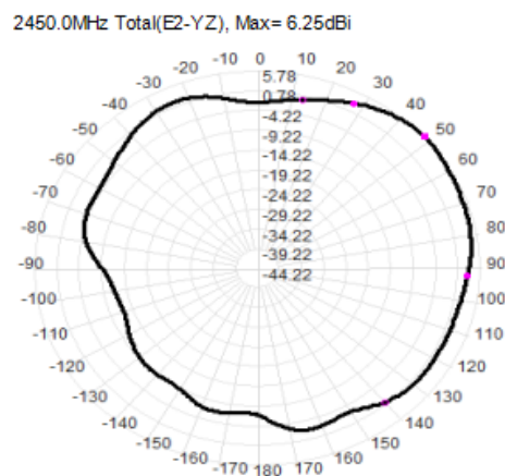
图 5 E2 面-总的增益方向图 E2 plane - total gain pattern
