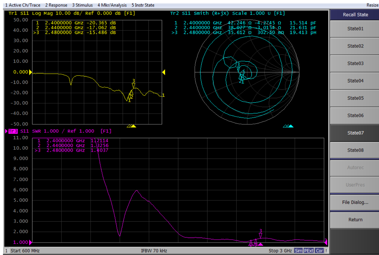
图 2 无源 S11 图 Passive S11 diagram
