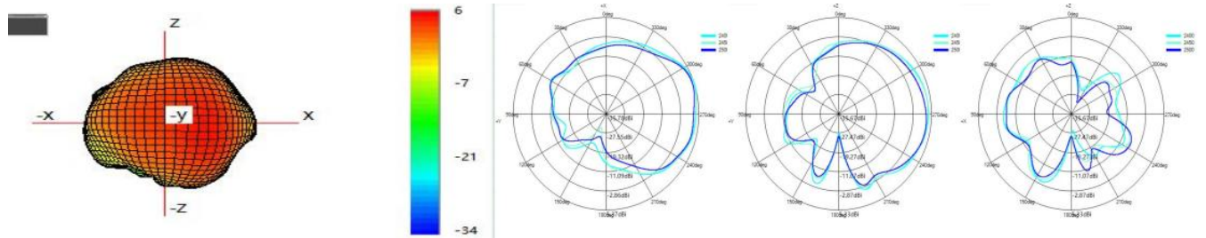
2450M 3D-E1-E2-H
