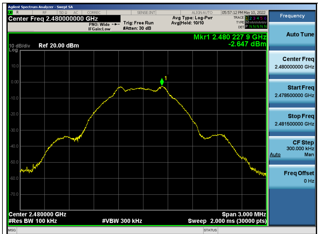
Test_Graph_2.4G_ANT1_2480_Reference Level
