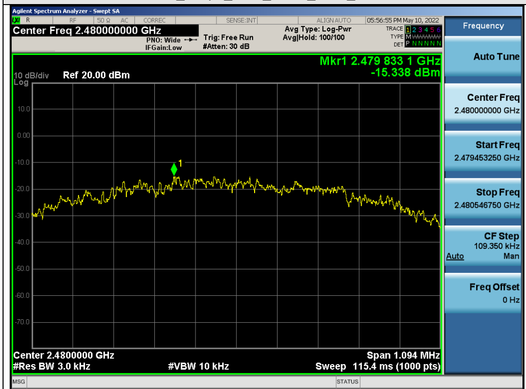
Test_Graph_2.4G_ANT1_2480_PSD
