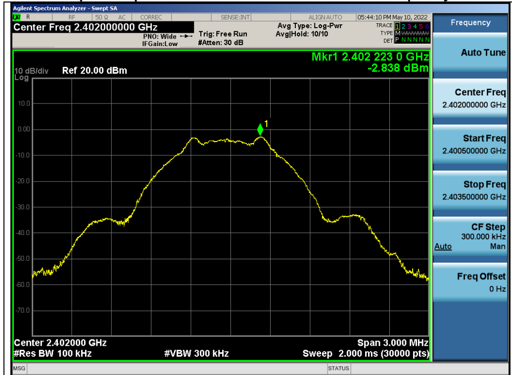
Test_Graph_2.4G_ANT1_2402_Reference Level
