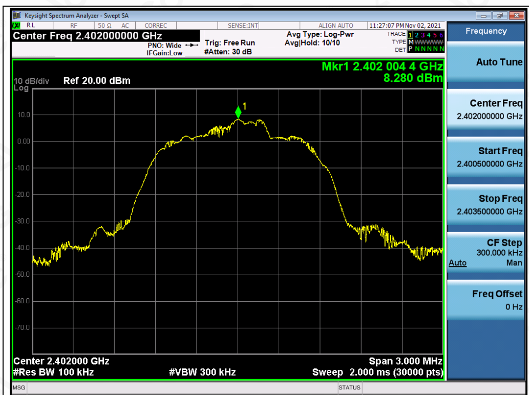
Test_Graph_EDR_ANT1_2402_3Mbps_Reference Level
