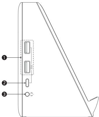
① USB-A 3.1 Gen 1 端口（5 Gbps，5V/0.9A）
