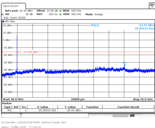
802.11b_2437MHz_Chain 0
