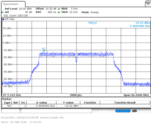
802.11n20_2412MHz_Chain 0
