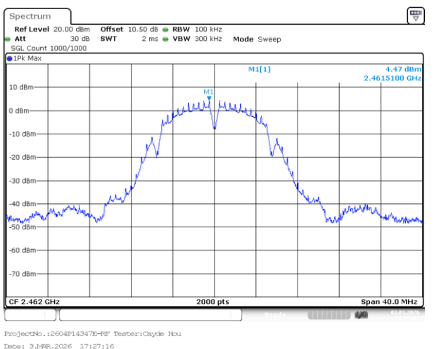
802.11b_2462MHz_Chain 0
