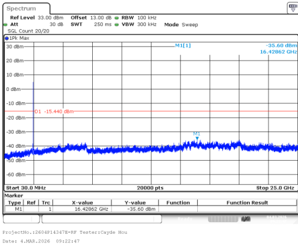
802.11b_2462MHz_Chain 1
