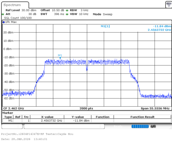
802.11n20_2462MHz_Chain 1
