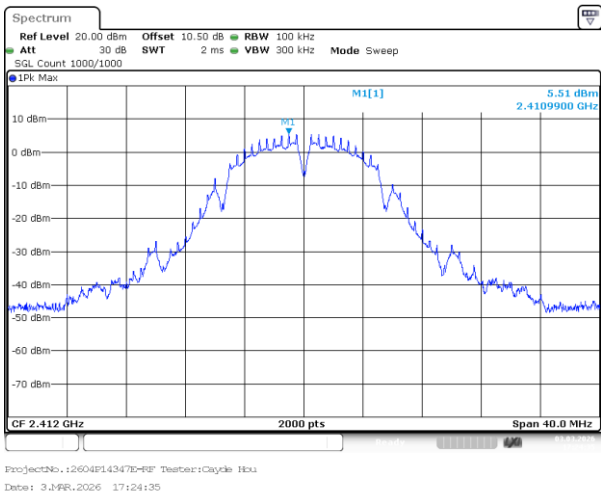
802.11b_2412MHz_Chain 0
