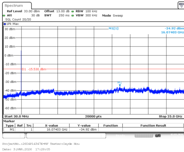
802.11b_2462MHz_Chain 0
