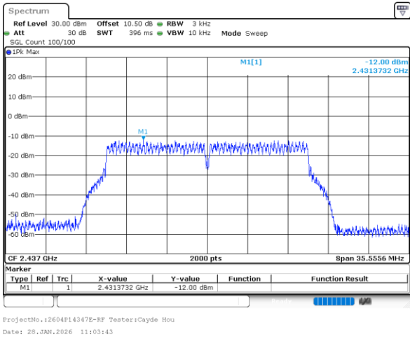
802.11n20_2437MHz_Chain 0
