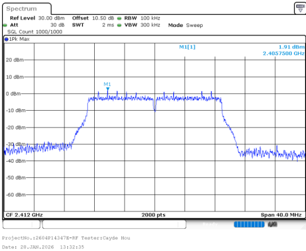
802.11n20_2412MHz_Chain 1
