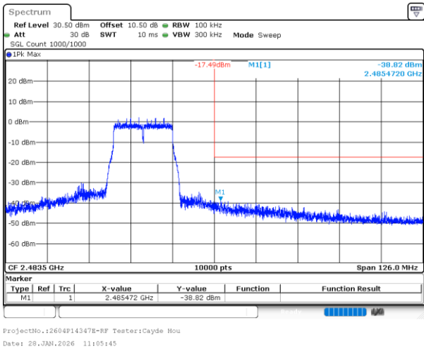
802.11n20_2462MHz_Chain 0
