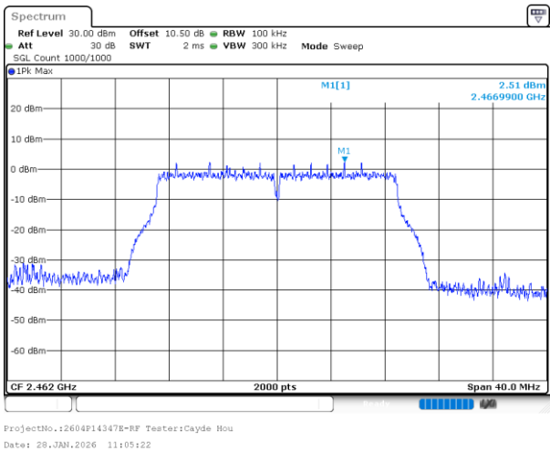
802.11n20_2462MHz_Chain 0
