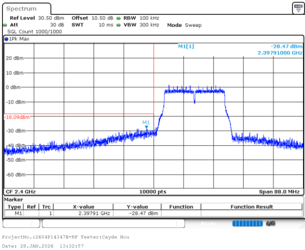
802.11n20_2412MHz_Chain 1
