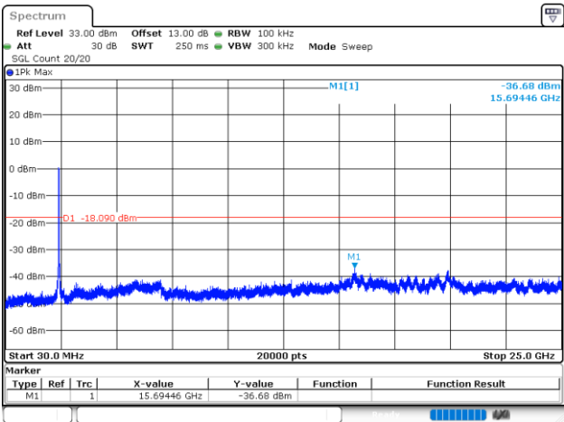
802.11n20_2412MHz_Chain 1
