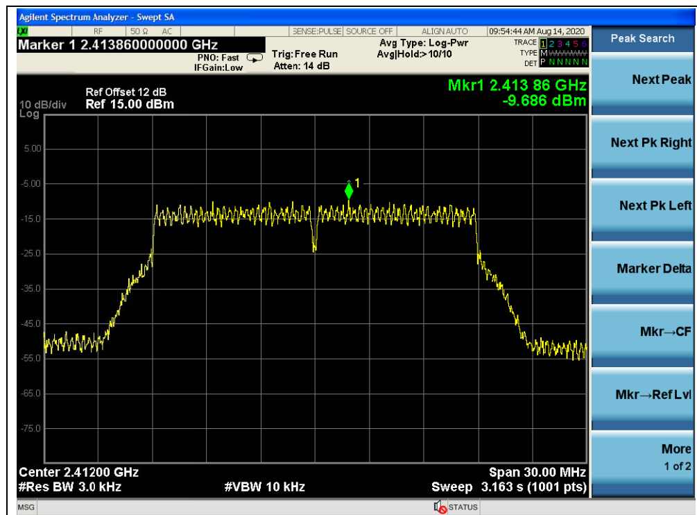
(Channel 1, 802.11n(HT20), ANT R)
