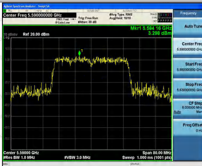
11N40SISO_Ant2_5590
