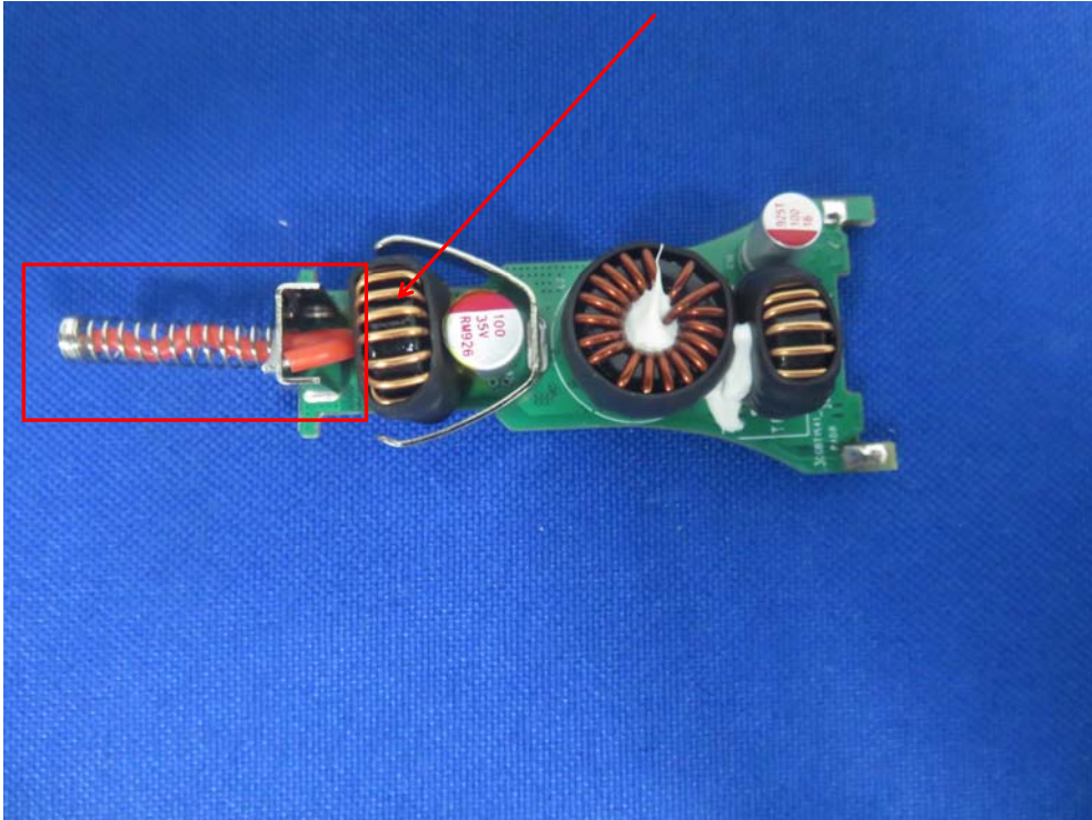
FM ANT
