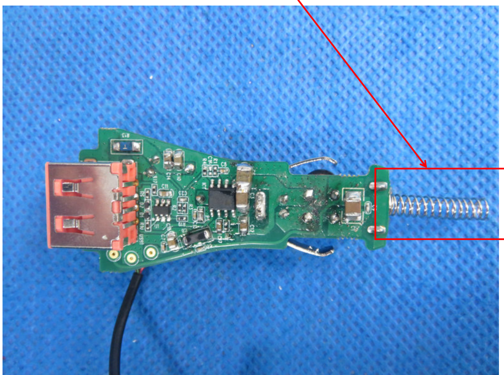
FM ANT
