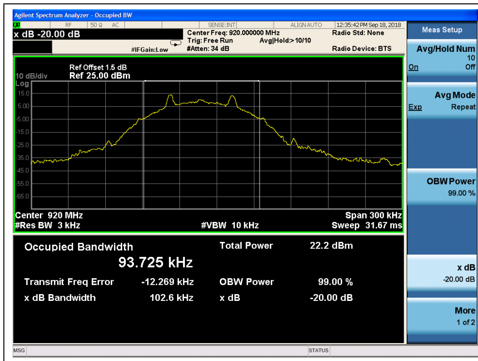
(Channel 1, 920.0MHz)
