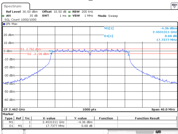
802.11n20_2462MHz
