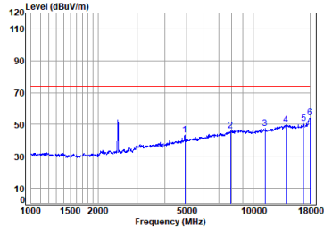
11n_20M_TX_CH_11_Horizontal-Peak
