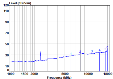
11n_20M_TX_CH_01_Vertical-Avg
