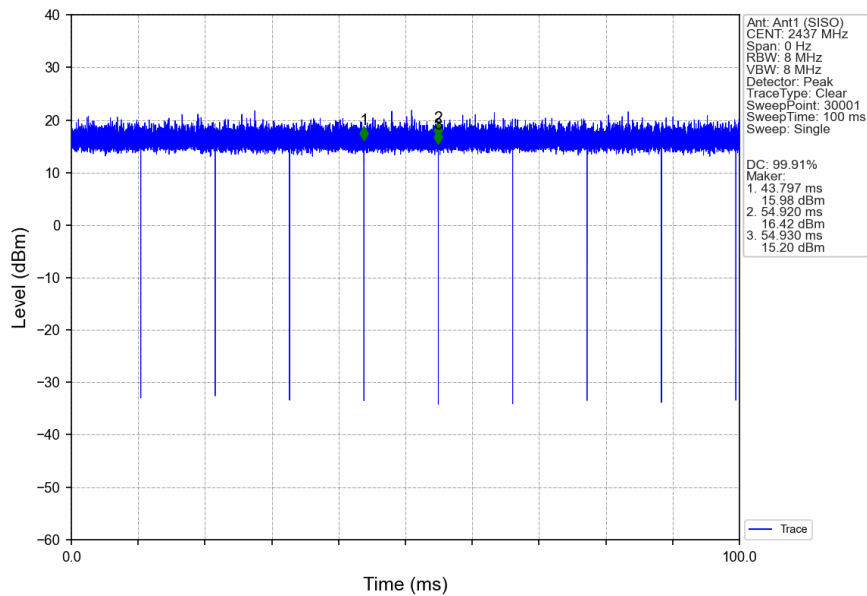
802.11n(HT20)_MCH_2437MHz_Ant1 (SISO)_NTNV
