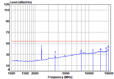
11n_20M_TX_CH_06_Horizontal-Avg
