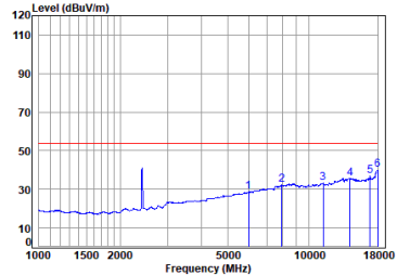
11n_20M_TX_CH_01_Horizontal-Avg
