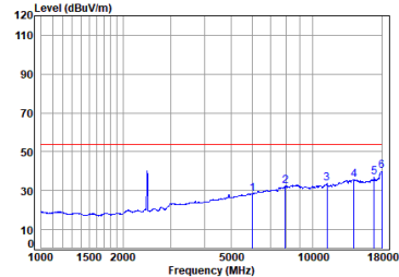
11g_TX_CH_11_Horizontal-Avg
