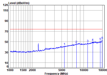
11n_20M_TX_CH_01_Vertical-Peak
