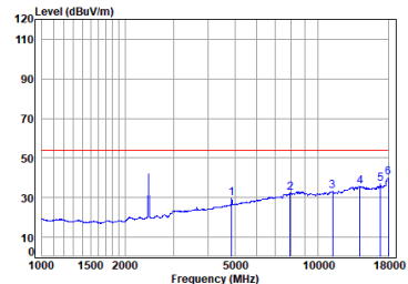
11n_20M_TX_CH_06_Vertical-Avg
