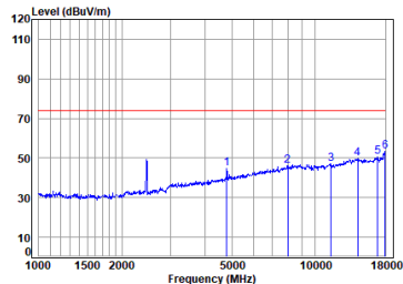
11n_20M_TX_CH_11_Vertical-Peak
