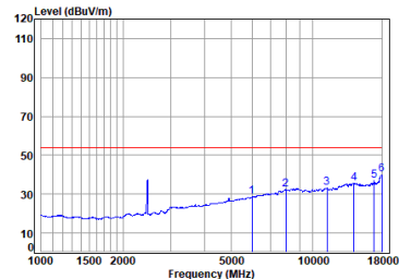
11g_TX_CH_11_Vertical-Avg
