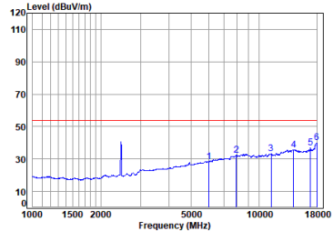
11n_20M_TX_CH_11_Horizontal-Avg
