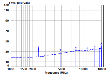
11g_TX_CH_01_Vertical-Avg
