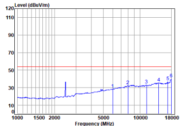
11n_20M_TX_CH_11_Vertical-Avg
