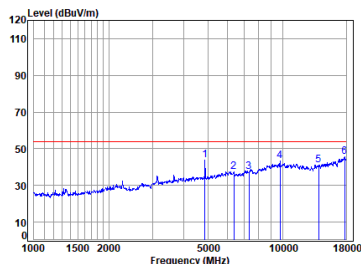
11b_TX_CH_06_Horizontal-Avg
