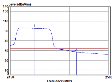
11g_TX_CH_11_Vertical-Avg
