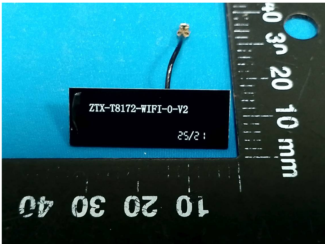
BLE&Wifi Antenna(Chain 0)
