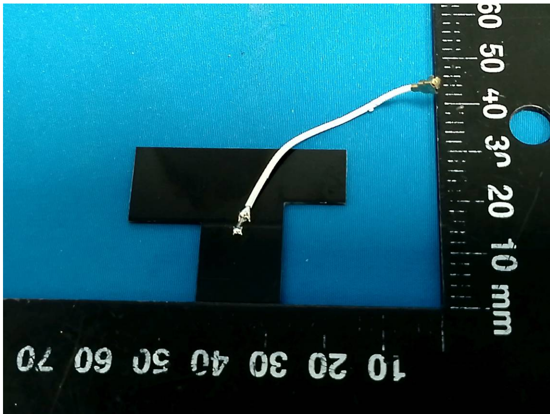
BLE&Wifi Antenna(Chain 0)
