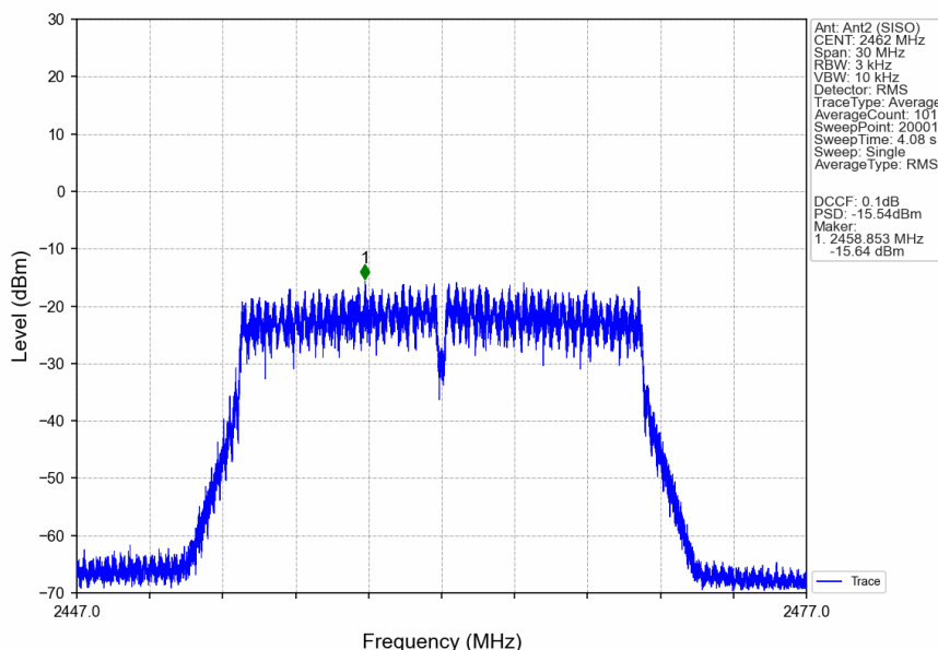
802.11g_HCH_2462MHz_Ant2 (SISO)_NTNV
