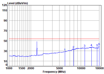
11n_20M_TX_CH_06_Horizontal-Avg
