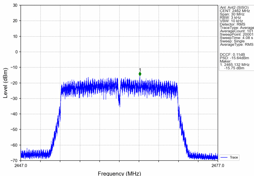
802.11n(HT20)_HCH_2462MHz_Ant2 (SISO)_NTNV
