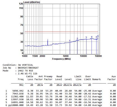
11b_TX_CH_11_Vertical-Avg
