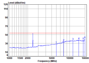
11b_TX_CH_06_Horizontal-Avg
