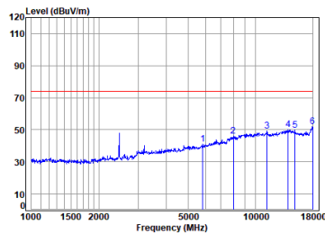
11n_20M_TX_CH_11_Vertical-Peak
