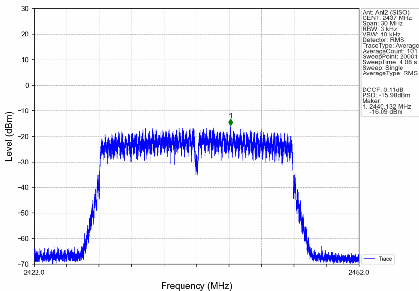
802.11n(HT20)_MCH_2437MHz_Ant2 (SISO)_NTNV
