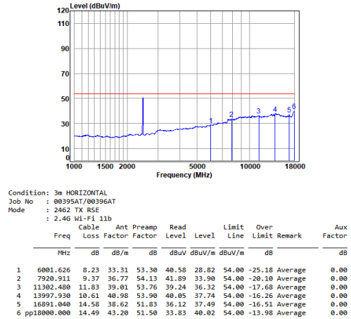
11b_TX_CH_11_Horizontal-Avg
