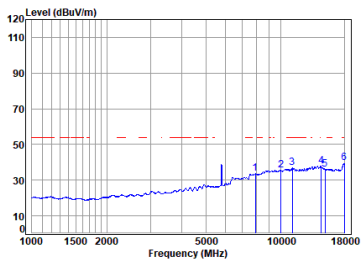
11ax_20M_TX_CH_157_Horizontal-Avg
