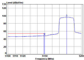
11ax_20M_TX_CH_36_Vertical-Avg
