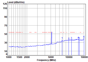
11ax_20M_TX_CH_36_Vertical-Avg
