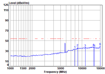
11a_TX_CH_157_Horizontal-Avg
