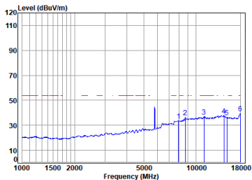
11ax_20M_TX_CH_157_Vertical-Avg
