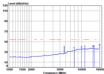
11ax_20M_TX_CH_149_Horizontal-Avg
