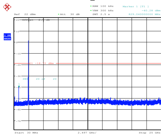
802.11b_2437MHz
