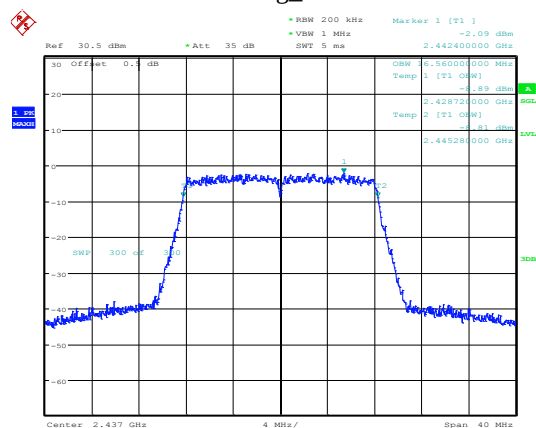
802.11g_2437MHz
