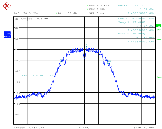
802.11b_2437MHz
