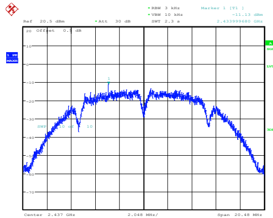
802.11b_2437MHz
