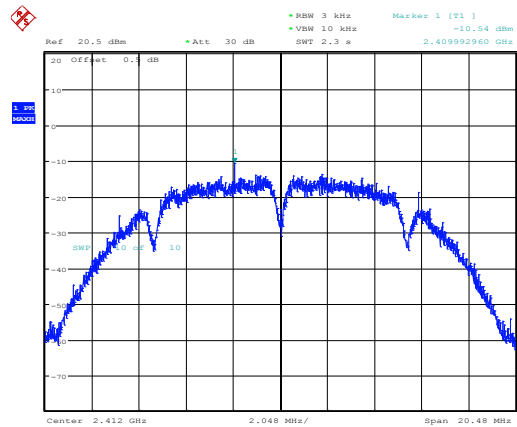
802.11b_2412MHz
