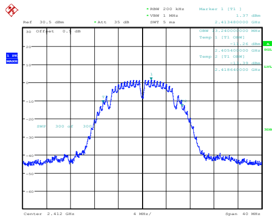
802.11b_2412MHz
