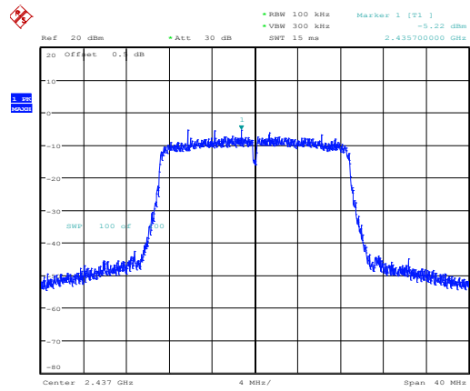
802.11n20_2437MHz
