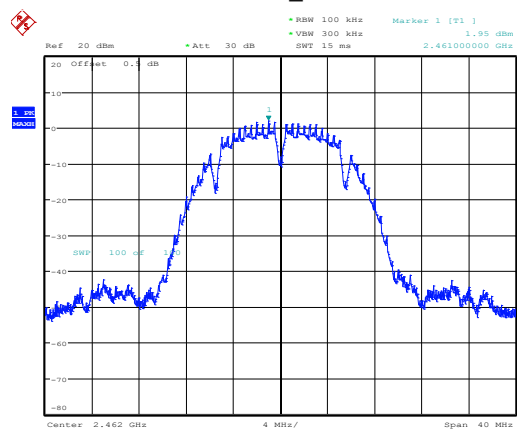
802.11b_2462MHz
