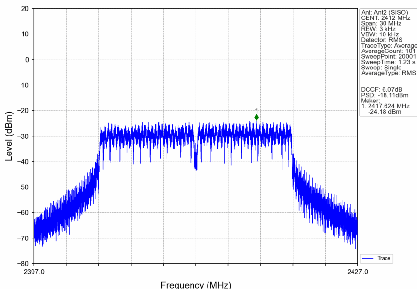
802.11n(HT20)_LCH_2412MHz_Ant2 (SISO)_NTNV
