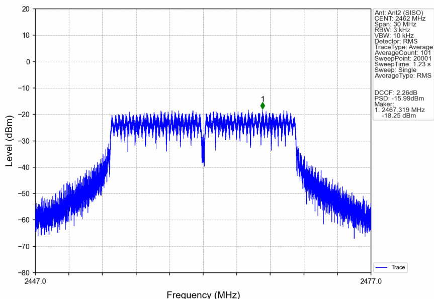
802.11g_HCH_2462MHz_Ant2 (SISO)_NTNV
