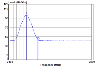
Antenna 1 BLE_2M_TX_CH_39_Vertical-Avg
