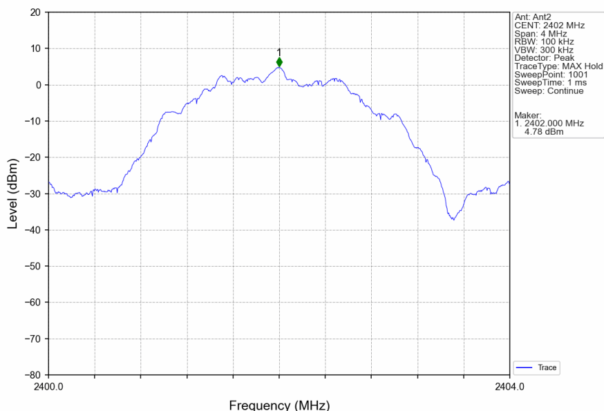
2M_LCH_2402MHz_Ant2_NTNV
