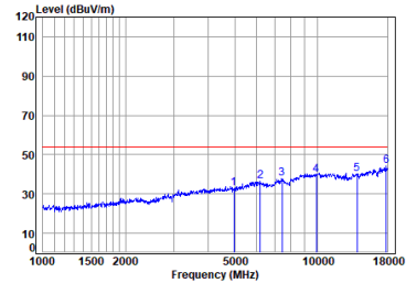
Antenna 0 BLE_2M_TX_CH_39_Horizontal-Avg
