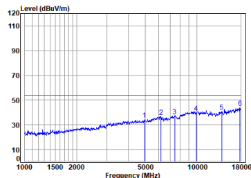
Antenna 1 BLE_2M_TX_CH_39_Horizontal-Avg
