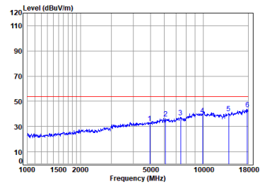
Antenna 0 BLE_2M_TX_CH_39_Vertical-Avg
