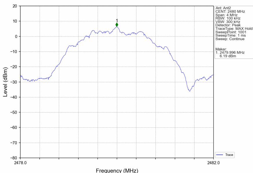
2M_HCH_2480MHz_Ant2_NTNV
