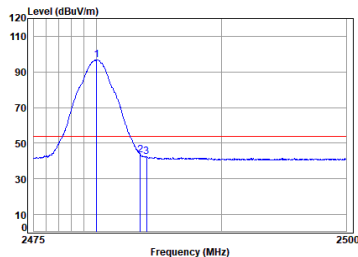
Antenna 0 BLE_2M_TX_CH_39_Vertical-Avg
