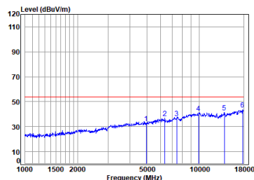
Antenna 1 BLE_2M_TX_CH_39_Vertical-Avg
