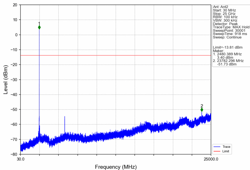
2M_HCH_2480MHz_Ant2_NTNV
