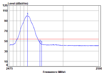
Antenna 0 BLE_2M_TX_CH_39_Horizontal-Avg
