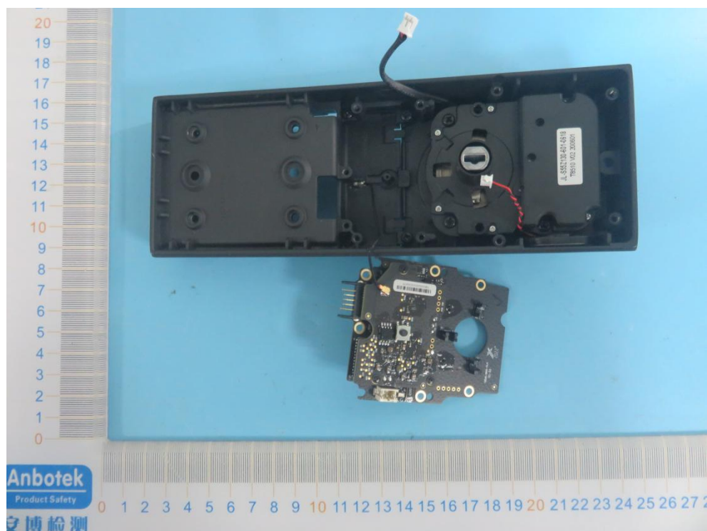
BT&WiFi ANT
