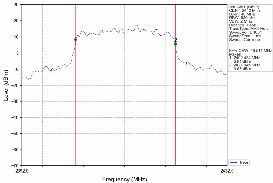
802.11ax(HEW20)_LCH_2412MHz_RU242_Left_Ant1 (SISO)_NTNV
