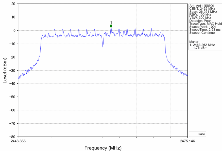
802.11ax(HEW20)_HCH_2462MHz_RU242_Left_Ant1 (SISO)_NTNV
