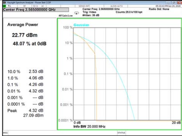
Band41_1_Q16_Low
