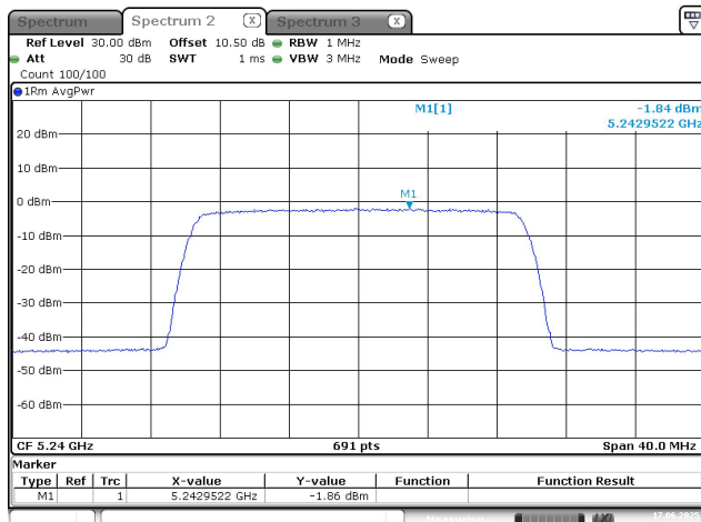
20M_5240MHz_Chain 0
