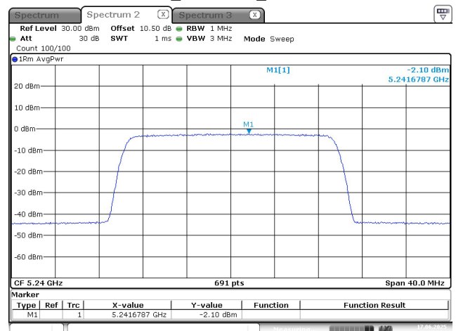
20M_5240MHz_Chain 1
