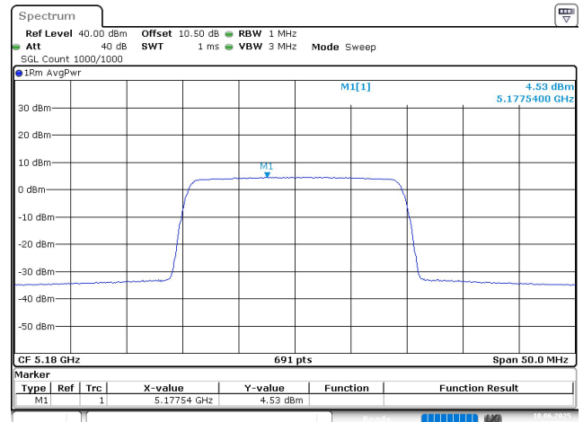
20M_5180MHz_Chain 1
