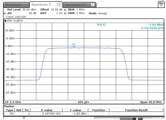
20M_5200MHz_Chain 0
