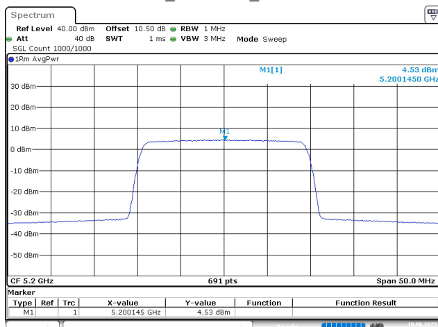
20M_5200MHz_Chain 1
