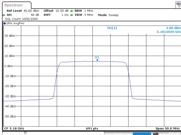
20M_5180MHz_Chain 0
