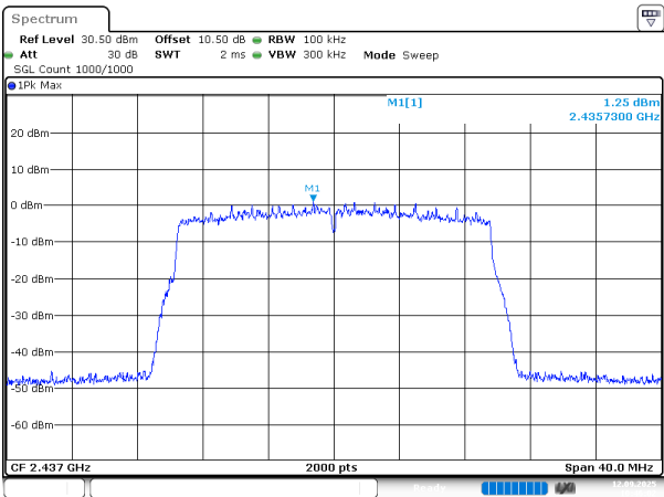
802.11ax20_2437MHz_Chain 0
