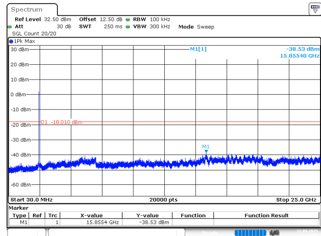
802.11ax20_2437MHz_Chain 1
