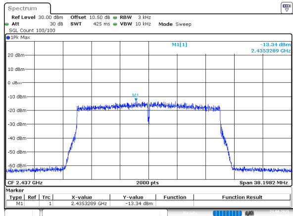
802.11ax20_2437MHz_Chain 1
