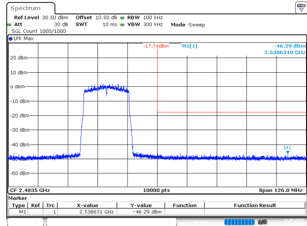
802.11ax20_2462MHz_Chain 1
