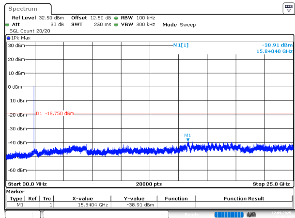
802.11ax20_2437MHz_Chain 0
