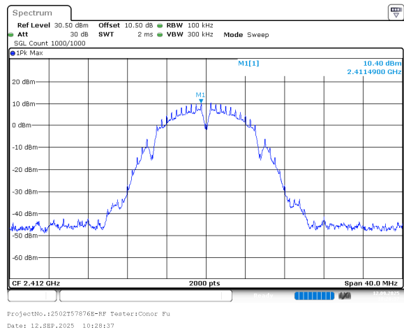
802.11b_2412MHz_Chain 0
