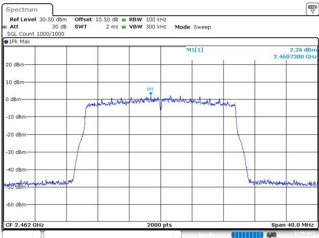
802.11ax20_2462MHz_Chain 1
