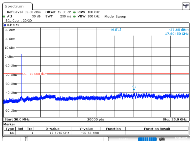
802.11ax20_2462MHz_Chain 0
