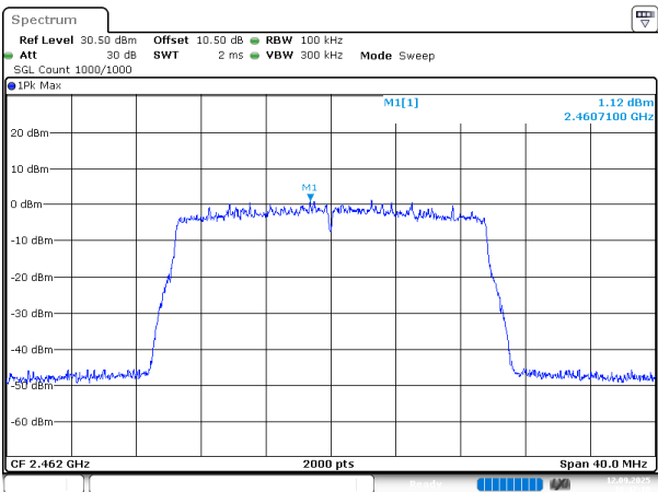
802.11ax20_2462MHz_Chain 0
