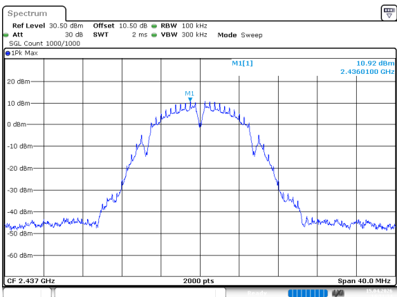
802.11b_2437MHz_Chain 0
