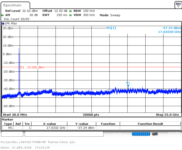
802.11n20_2412MHz_Chain 0
