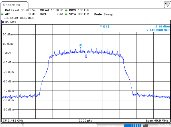
802.11n20_2412MHz_Chain 1
