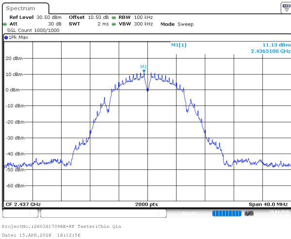
802.11b_2437MHz_Chain 1
