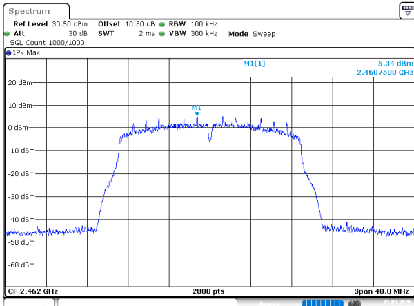
802.11n20_2462MHz_Chain 0
