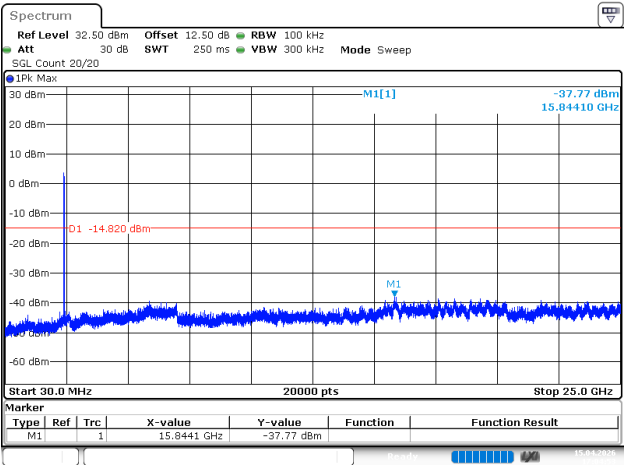
802.11n20_2412MHz_Chain 1
