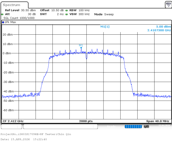
802.11n20_2412MHz_Chain 0
