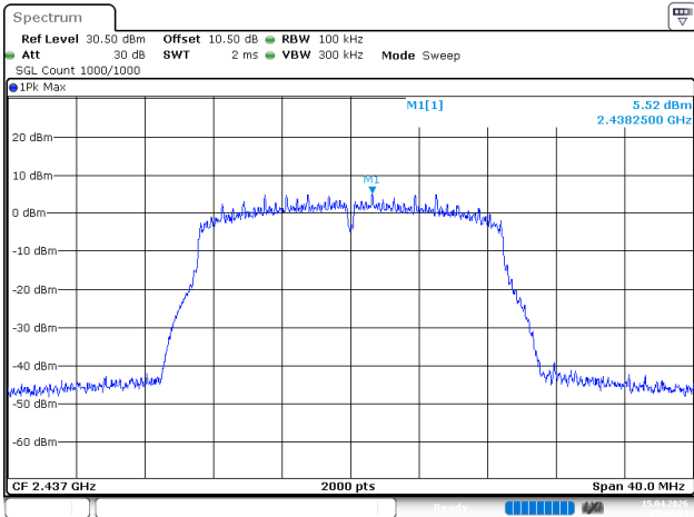
802.11n20_2437MHz_Chain 1
