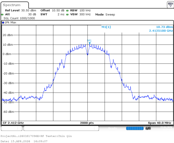
802.11b_2412MHz_Chain 1
