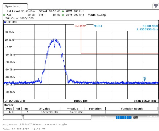
802.11b_2462MHz_Chain 1
