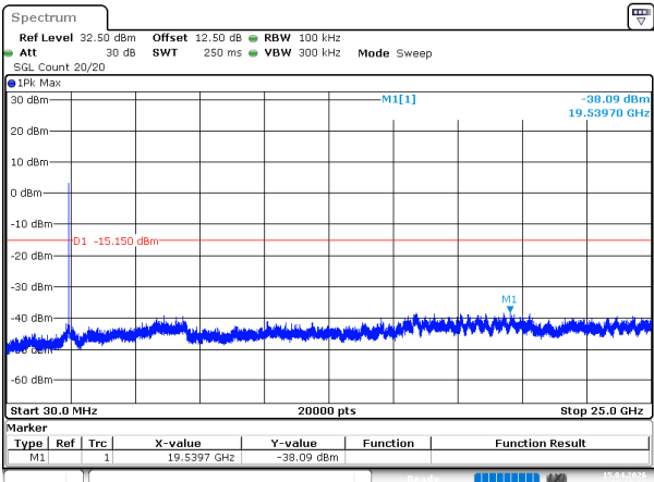
802.11n20_2437MHz_Chain 0
