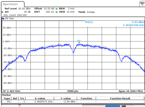
802.11b_2462MHz_Chain 1
