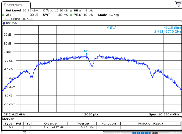
802.11b_2412MHz_Chain 1
