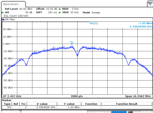
802.11b_2437MHz_Chain 0
