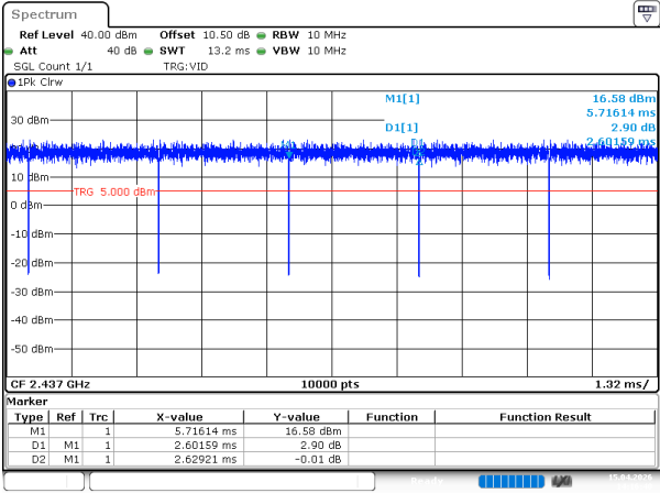
802.11n20_2437MHz_Chain 0
