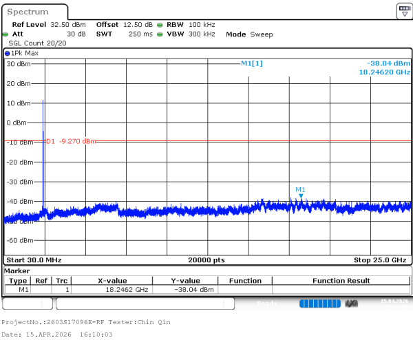
802.11b_2412MHz_Chain 1
