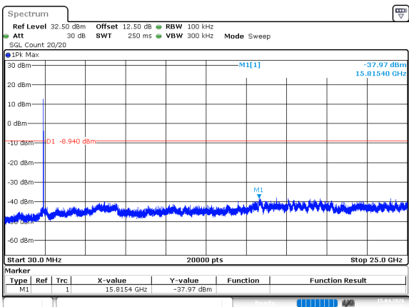
802.11b_2412MHz_Chain 0
