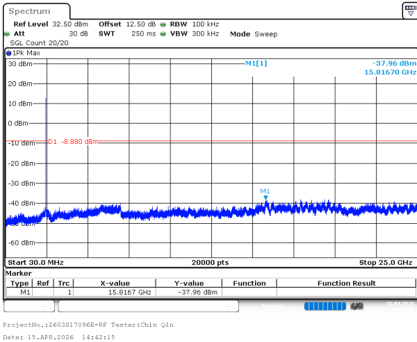
802.11b_2462MHz_Chain 0
