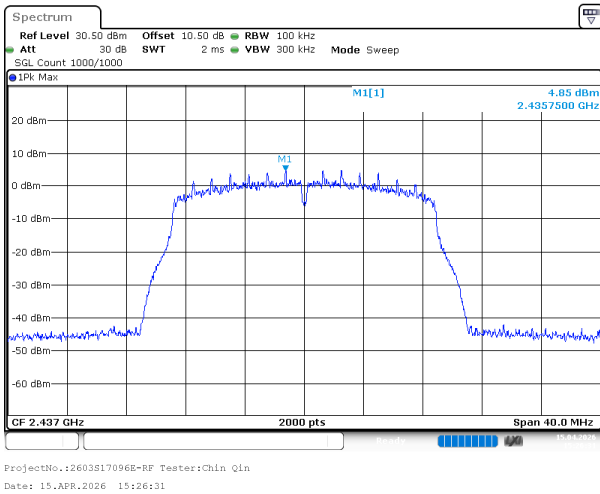
802.11n20_2437MHz_Chain 0
