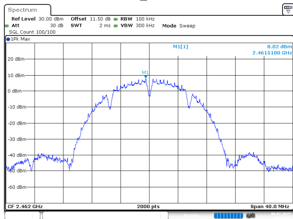
802.11b_2462MHz
