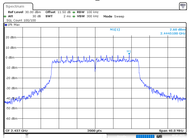
802.11ax20_2437MHz
