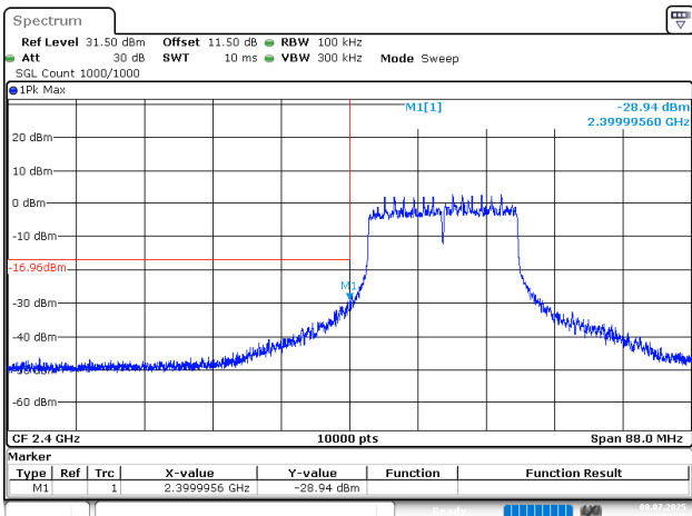
802.11ax20_2412MHz
