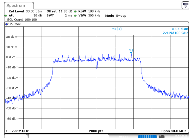
802.11ax20_2412MHz
