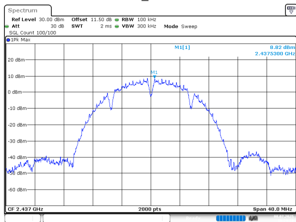
802.11b_2437MHz
