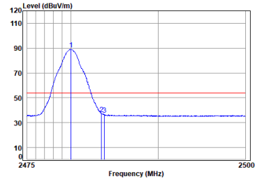
antenna 0 BLE_2M_TX_CH_39_Horizontal-Avg
