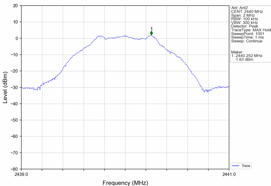
1M_MCH_2440MHz_Ant2_NTNV
