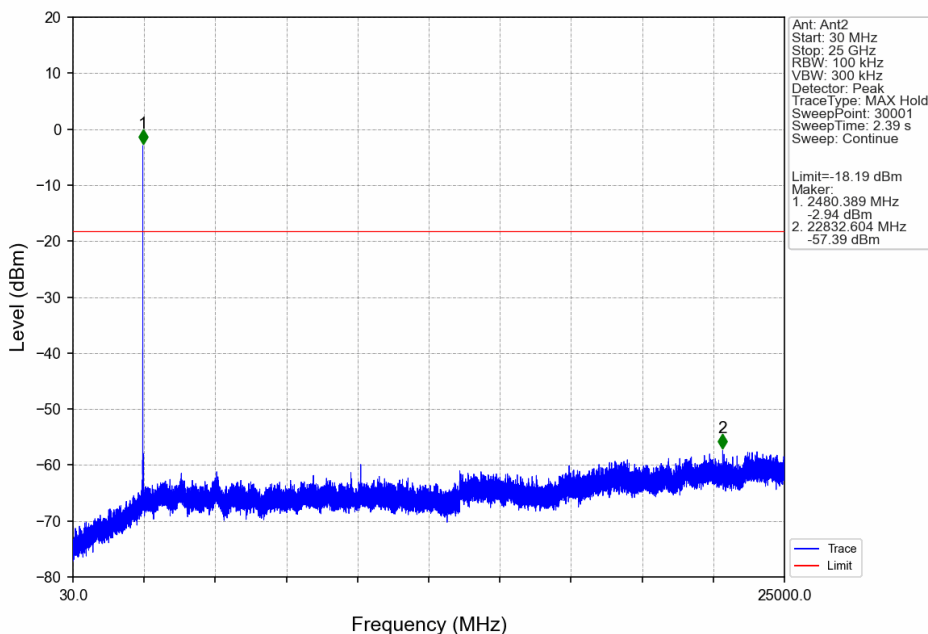
2M_HCH_2480MHz_Ant2_NTNV
