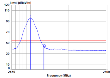
antenna 0 BLE_2M_TX_CH_39_Vertical-Avg
