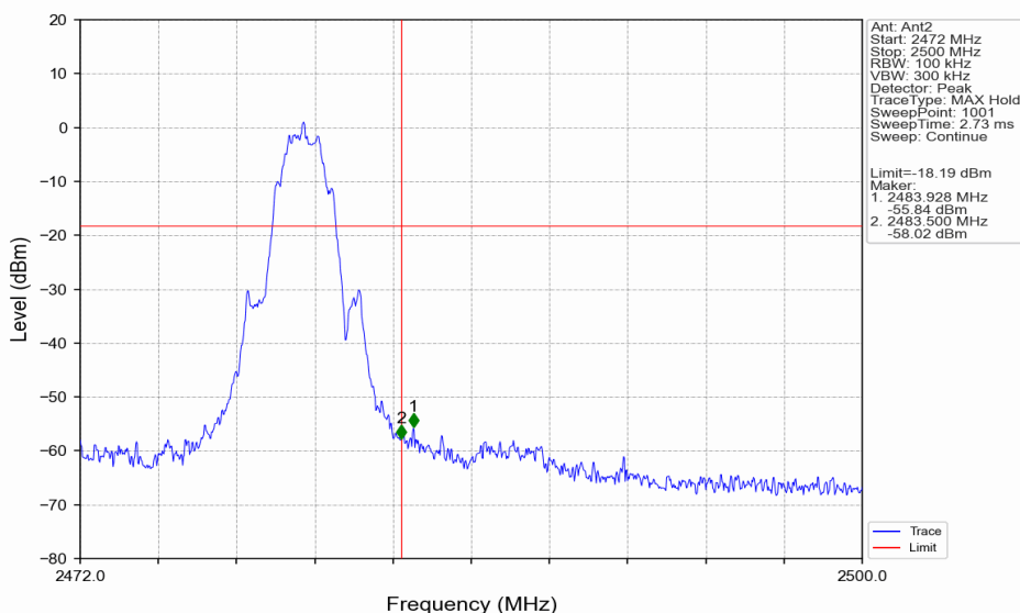
2M_HCH_2480MHz_Ant2_NTNV
