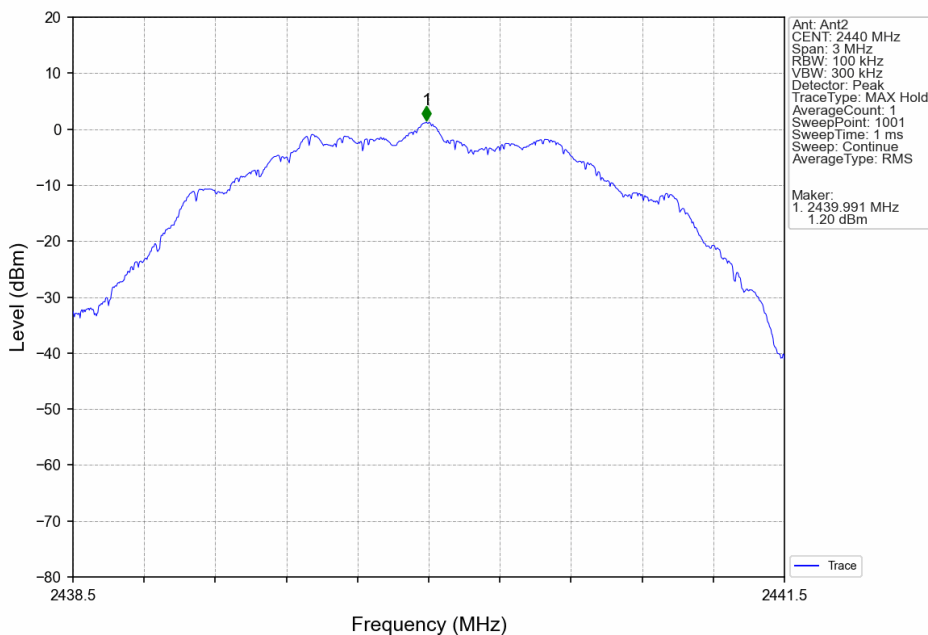
2M_MCH_2440MHz_Ant2_NTNV
