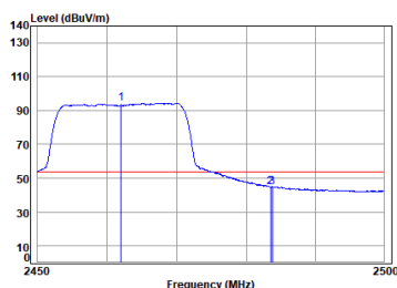
antenna 1 11n_HT(20M)_TX_CH_11_Vertical-Avg
