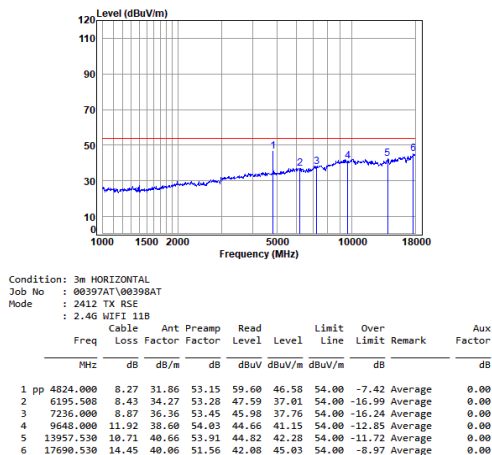
antenna 0 11b_TX_CH_01_Horizontal-Avg
