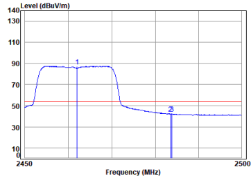
antenna 0 11g_TX_CH_11_Horizontal-Avg
