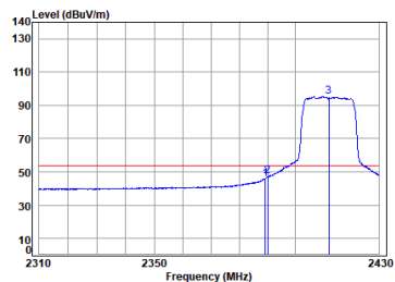
antenna 1 11n_HT(20M)_TX_CH_01_Vertical-Avg
