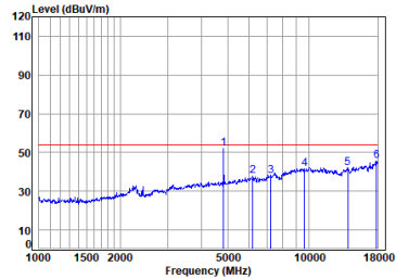
antenna 1 11b_TX_CH_01_Horizontal-Avg
