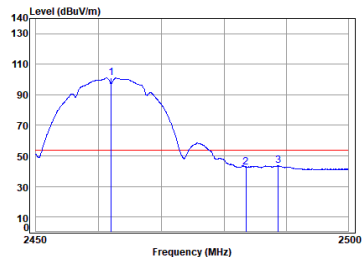
antenna 1 11b_TX_CH_11_Vertical-Avg
