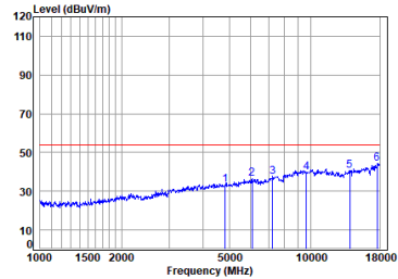
antenna 0 11n_HT(20M)_TX_CH_01_Horizontal-Avg
