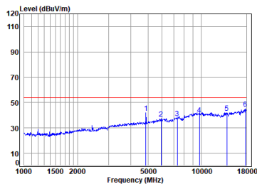
antenna 0 11b_TX_CH_06_Horizontal-Avg
