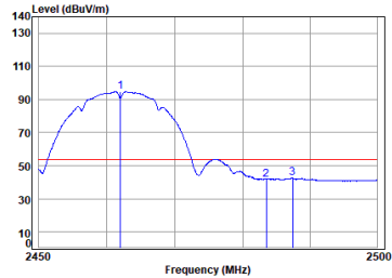
antenna 0 11b_TX_CH_11_Horizontal-Avg
