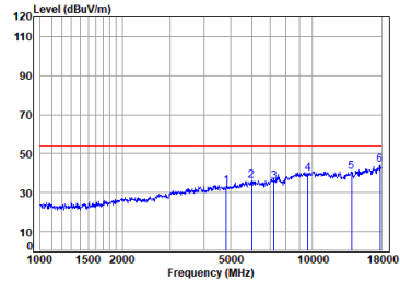
antenna 1 11n_HT(20M)_TX_CH_01_Horizontal-Avg
