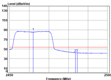
antenna 0 11n_HT(20M)_TX_CH_11_Horizontal-Avg
