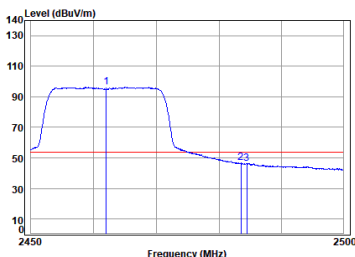
antenna 0 11n_HT(20M)_TX_CH_11_Vertical-Avg
