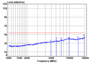
antenna 0 11n_HT(20M)_TX_CH_11_Vertical-Avg
