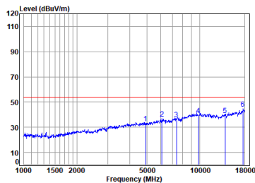
antenna 1 11n_HT(20M)_TX_CH_11_Horizontal-Avg
