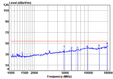
antenna 1 11b_TX_CH_06_Vertical-Avg
