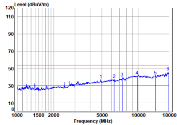
antenna 1 11b_TX_CH_11_Vertical-Avg
