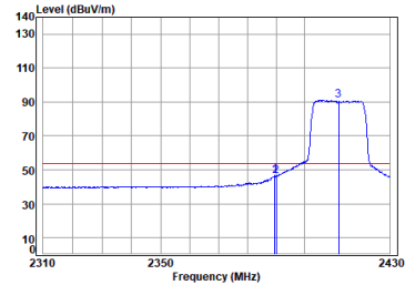
antenna 0 11n_HT(20M)_TX_CH_01_Horizontal-Avg
