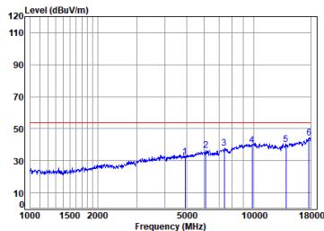
antenna 1 11n_HT(20M)_TX_CH_11_Vertical-Avg
