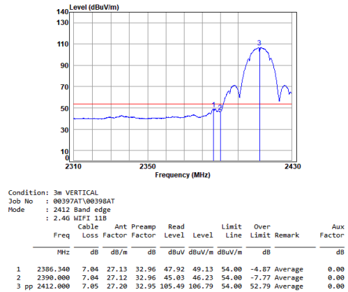
antenna 0 11b_TX_CH_01_Vertical-Avg
