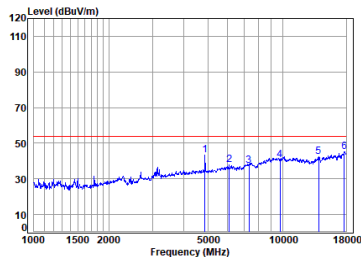
antenna 0 11b_TX_CH_06_Vertical-Avg
