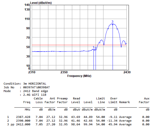
antenna 0 11b_TX_CH_01_Horizontal-Avg
