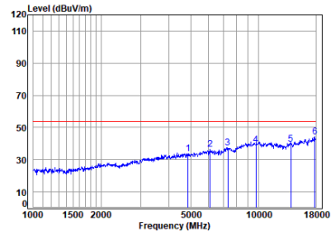
antenna 1 11n_HT(20M)_TX_CH_06_Vertical-Avg
