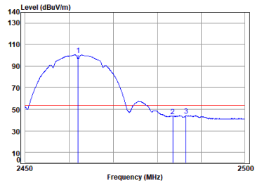
antenna 1 11b_TX_CH_11_Horizontal-Avg
