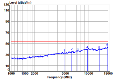
antenna 0 11n_HT(20M)_TX_CH_06_Horizontal-Avg
