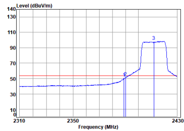
antenna 0 11n_HT(20M)_TX_CH_01_Vertical-Avg
