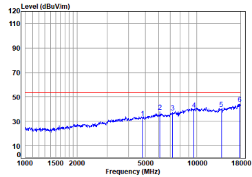
antenna 0 11n_HT(20M)_TX_CH_01_Vertical-Avg
