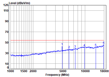
antenna 0 11b_TX_CH_11_Horizontal-Avg
