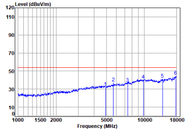
antenna 0 11n_HT(20M)_TX_CH_11_Horizontal-Avg
