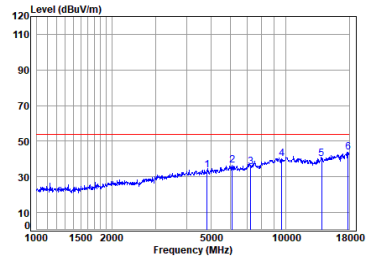
antenna 1 11n_HT(20M)_TX_CH_01_Vertical-Avg
