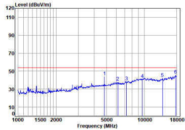
antenna 1 11b_TX_CH_01_Vertical-Avg
