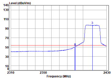
antenna 1 11n_HT(20M)_TX_CH_01_Horizontal-Avg
