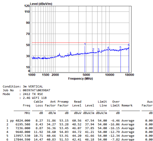
antenna 0 11b_TX_CH_01_Vertical-Avg
