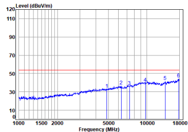
antenna 0 11n_HT(20M)_TX_CH_06_Vertical-Avg
