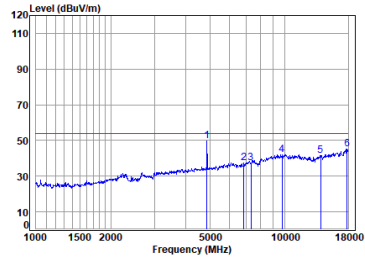
antenna 1 11b_TX_CH_06_Horizontal-Avg
