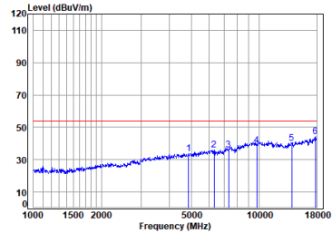
antenna 1 11n_HT(20M)_TX_CH_06_Horizontal-Avg
