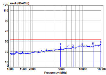
antenna 0 11b_TX_CH_11_Vertical-Avg
