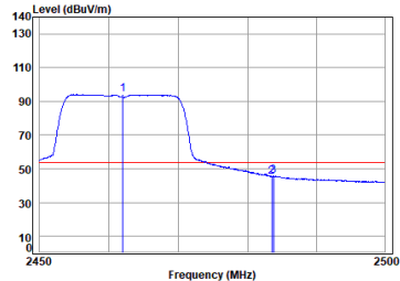
antenna 1 11g_TX_CH_11_Horizontal-Avg
