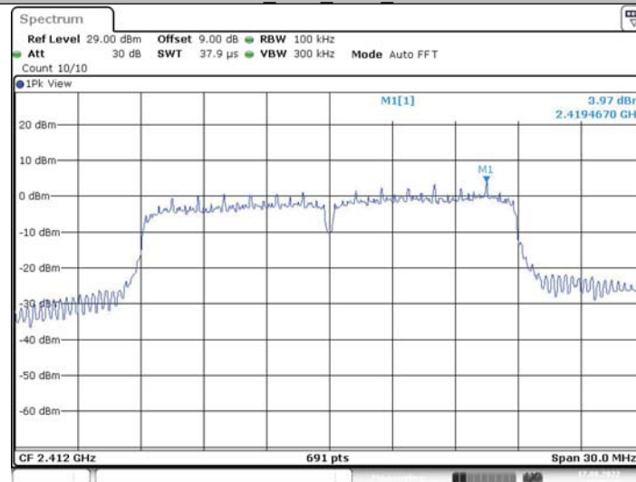
11N20MIMO_Ant2_2412_0~Reference
