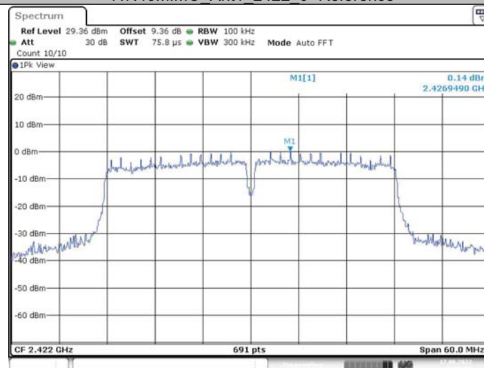
11N40MIMO_Ant1_2422_0~Reference
