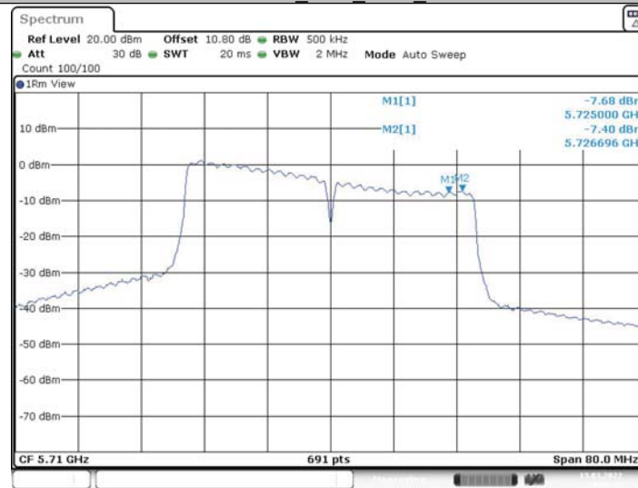
11N40MIMO_Ant2_5710_UNII-3
