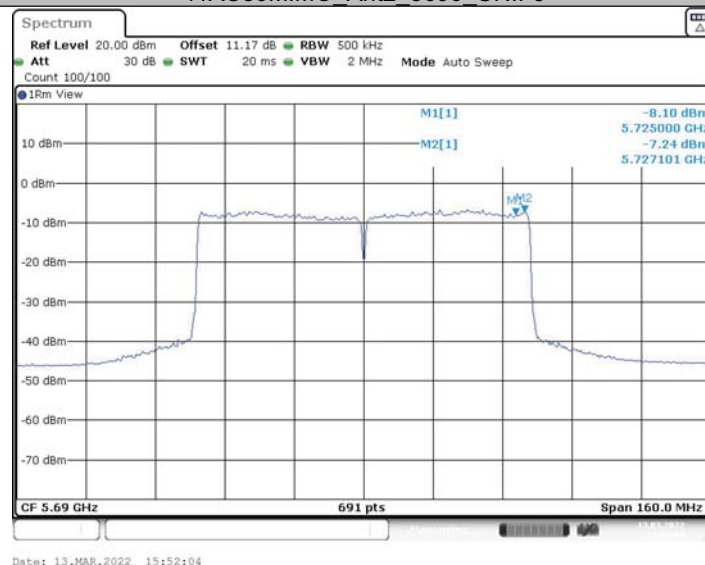
11AC80MIMO_Ant2_5690_UNII-3
