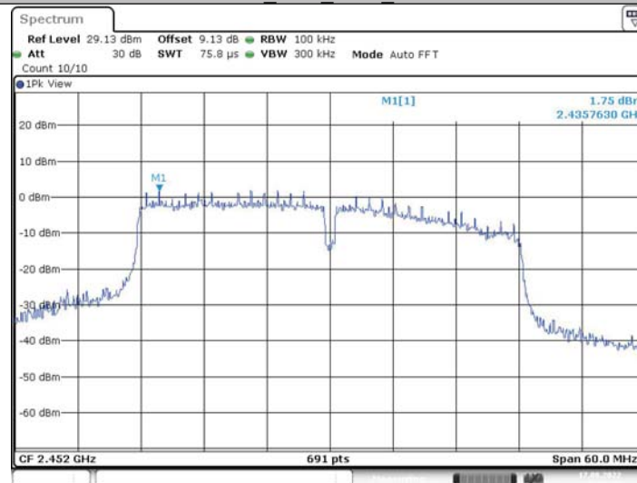
11N40MIMO_Ant2_2452_0~Reference
