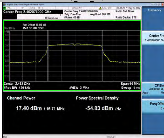
11G_Ant2_2462
