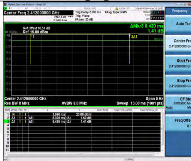
11B_Ant2_2412
