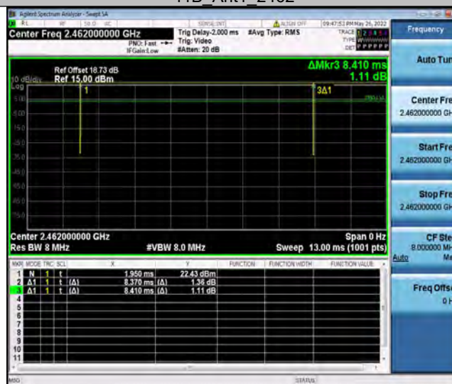
11B_Ant2_2462
