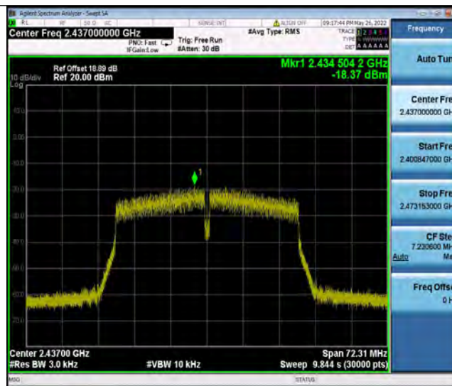
11N40SISO_Ant2_2437
