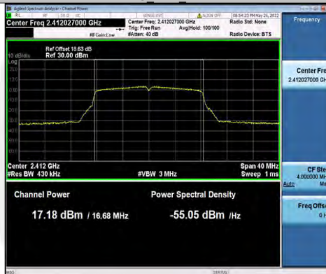
11G_Ant2_2412
