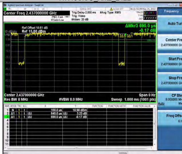
11N40SISO Ant1 2437
