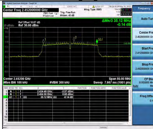
11N40SISO Ant1 2452
