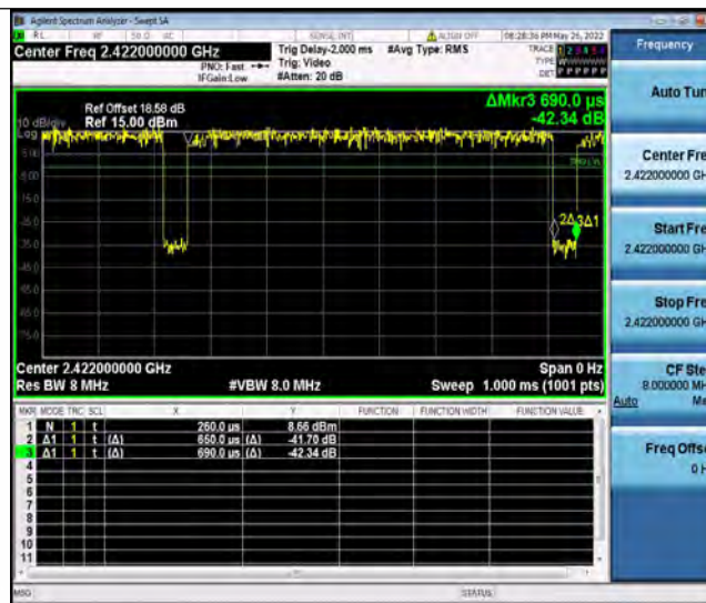
11N40SISO Ant1 2422
