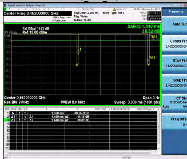
11G_Ant2_2462
