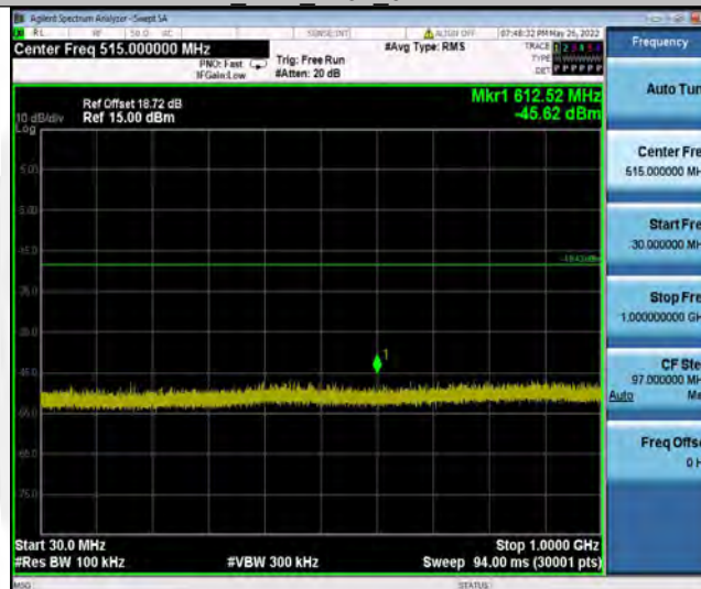
11B_Ant1_2462_30~1000
