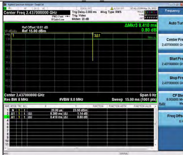
11B_Ant1_2437
