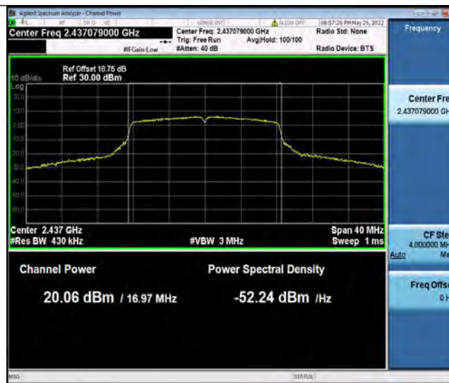
11G_Ant2_2437
