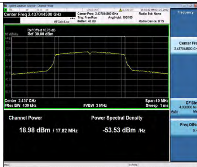
11N20SISO_Ant2_2437
