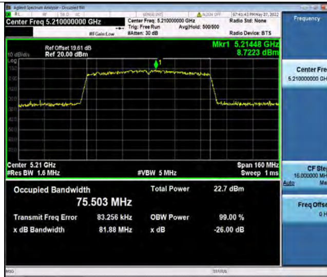
11AC80SISO_Ant1_5210
