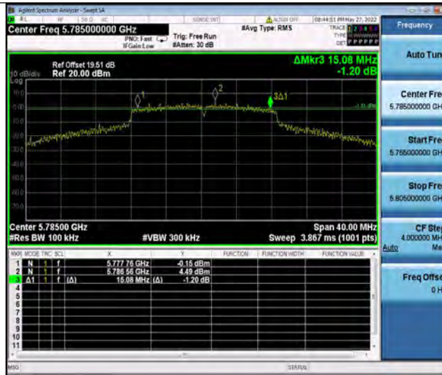
11A_Ant2_5785
