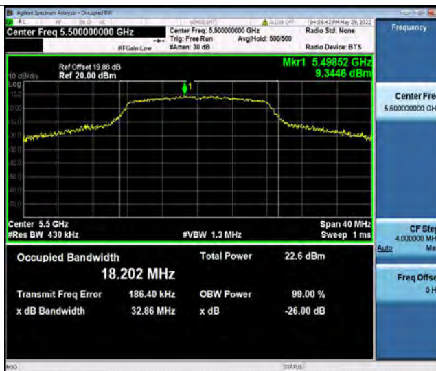
11A Ant1 5500
