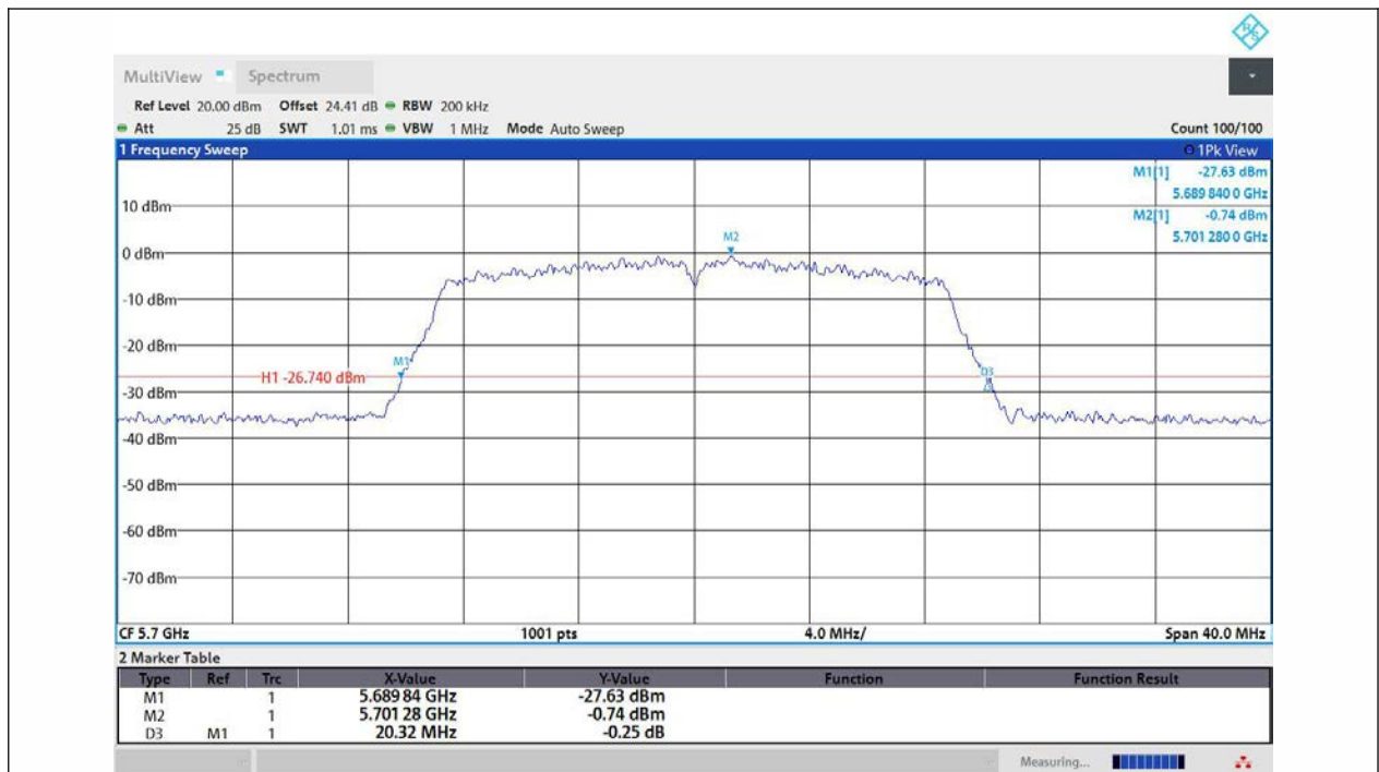
11N20MIMO-Ant1-5700
