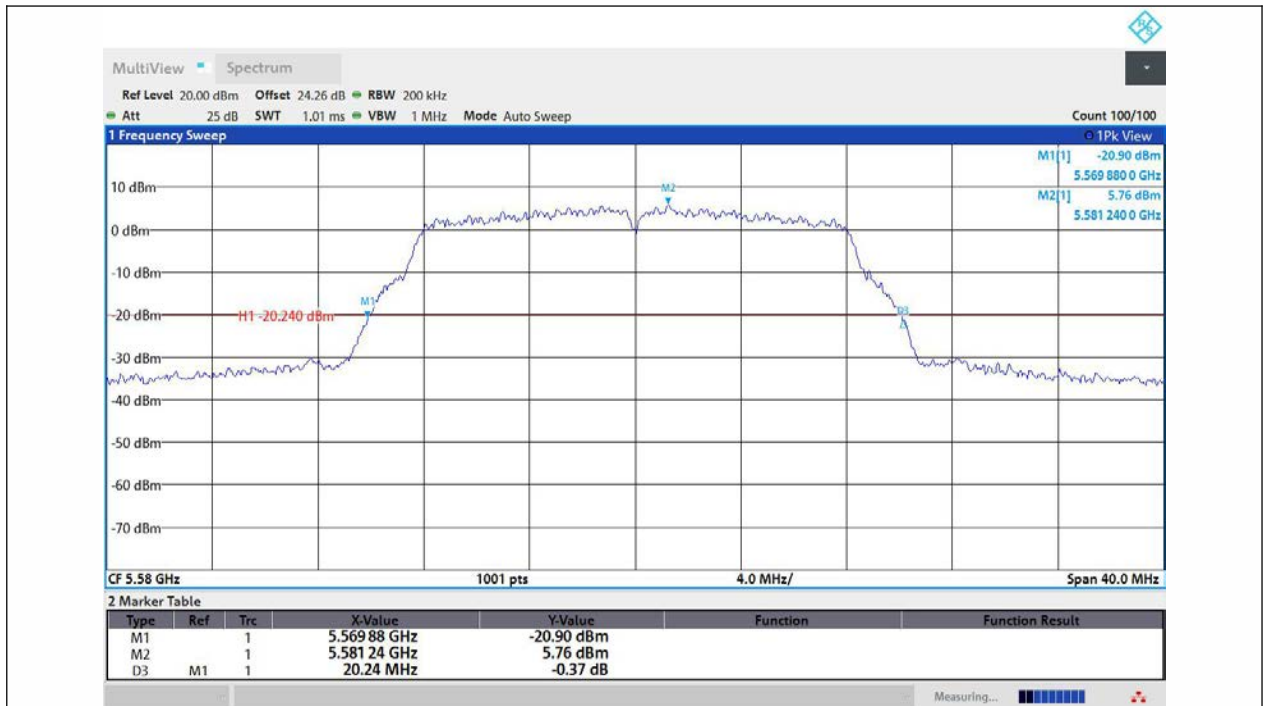
11A-Ant1-5580
