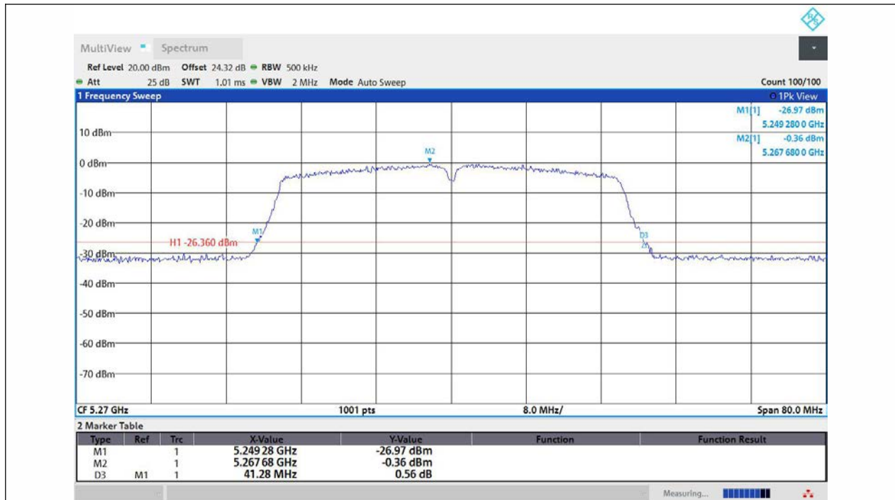
11AC40MIMO-Ant1-5270
