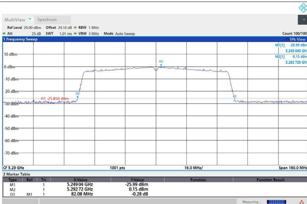
11AC80MIMO-Ant1-5290
