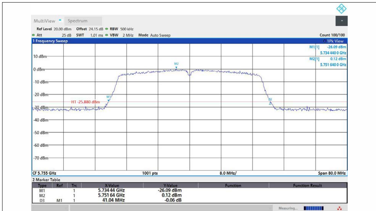
11AC40MIMO-Ant1-5755
