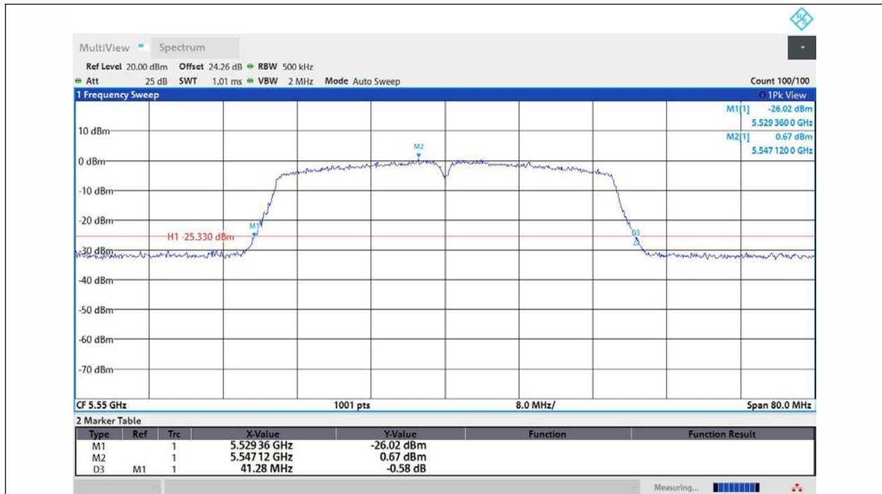
11AC40MIMO-Ant1-5550
