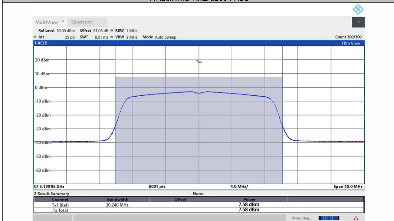
11N20MIMO-Ant1-5200-PASS
