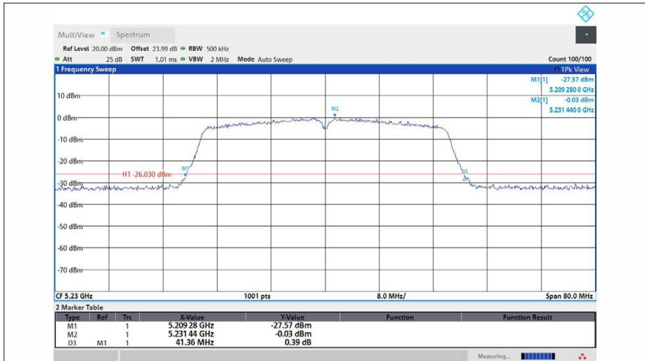
11AC40MIMO-Ant1-5230
