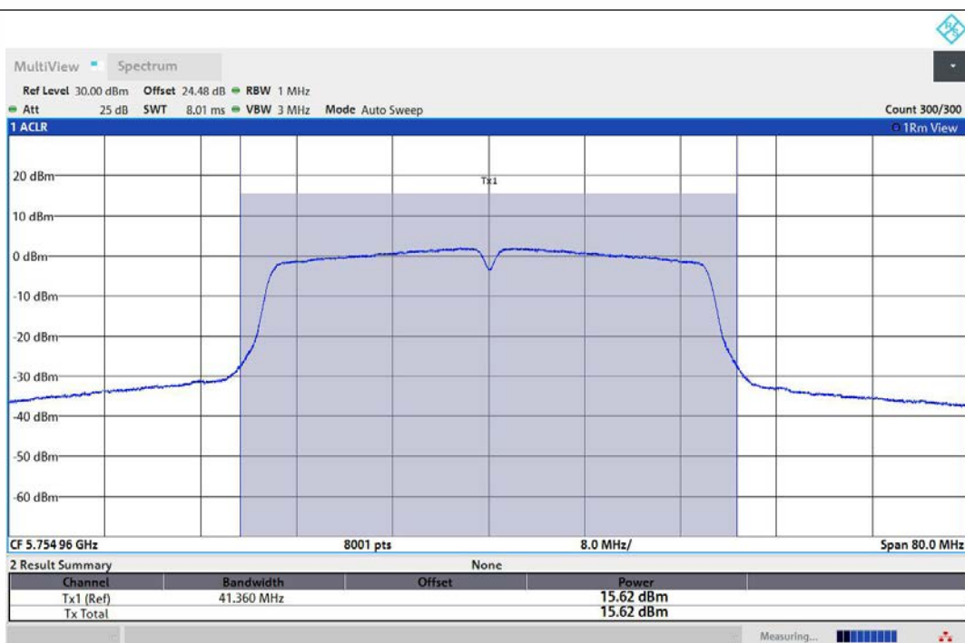
11N40MIMO-Ant1-5755-PASS
