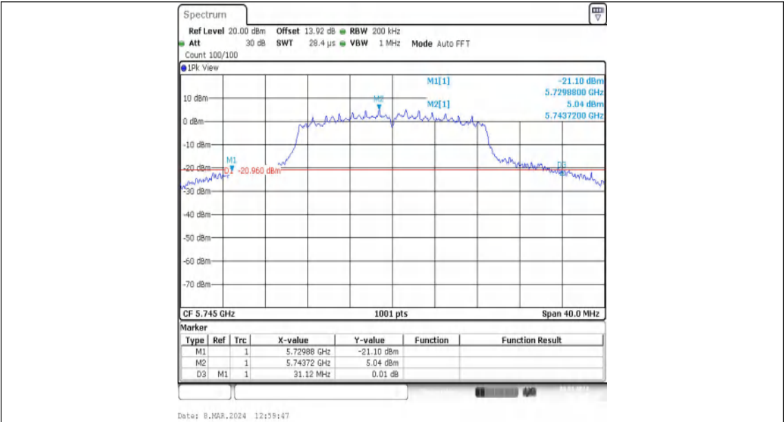
11N20MIMO-Ant1-5745
