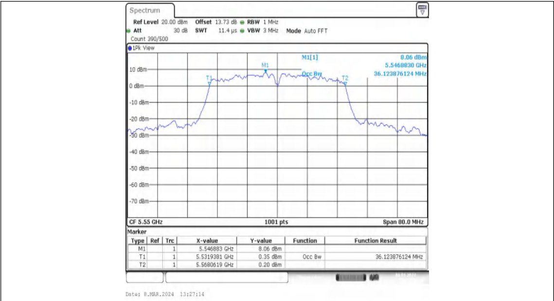
11N40MIMO-Ant1-5550
