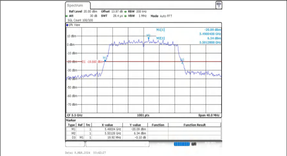
11N20MIMO-Ant2-5500
