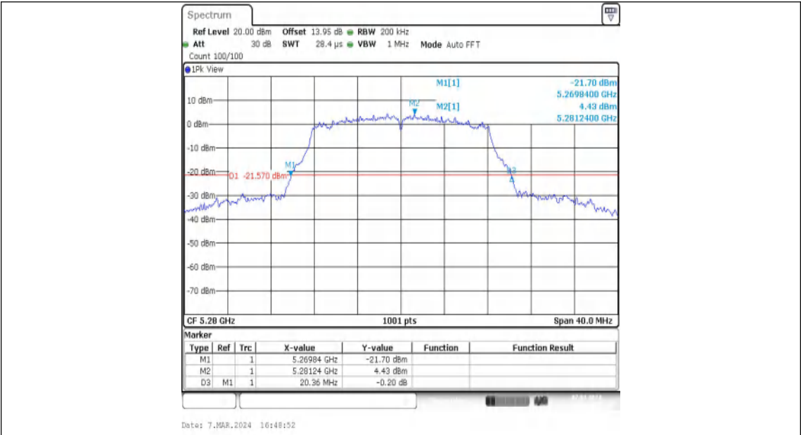
11A-Ant1-5280
