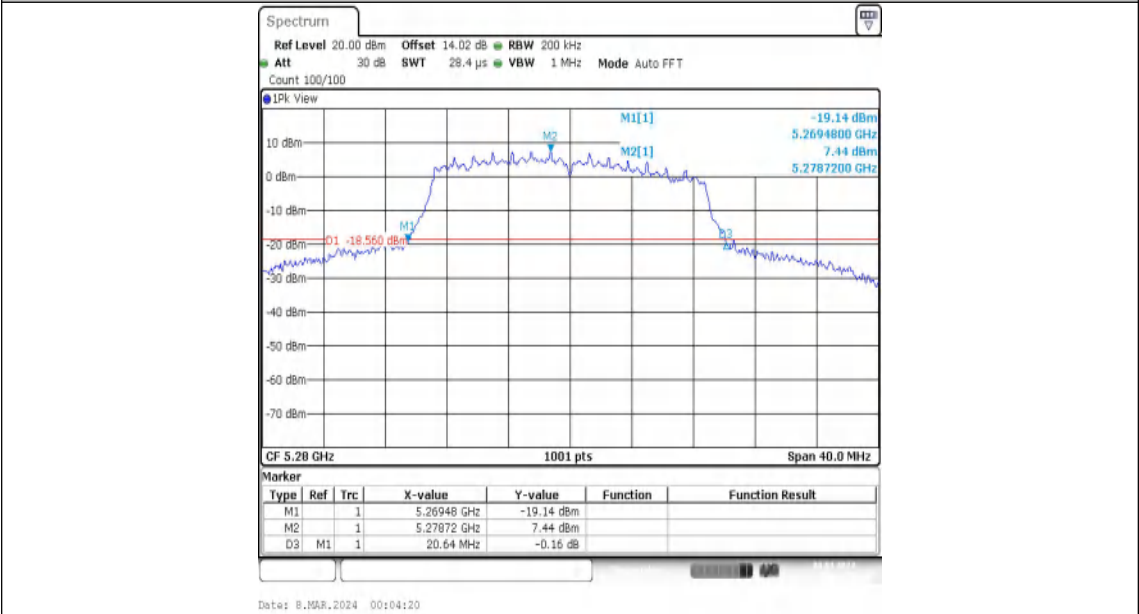
11N20MIMO-Ant2-5280
