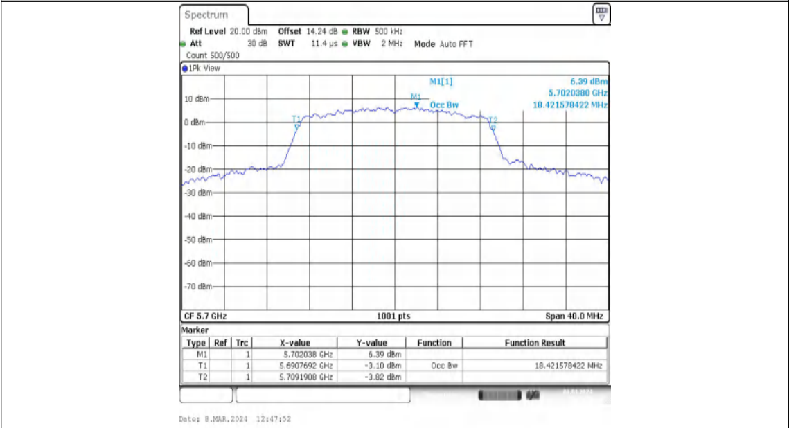
11N20MIMO-Ant2-5700
