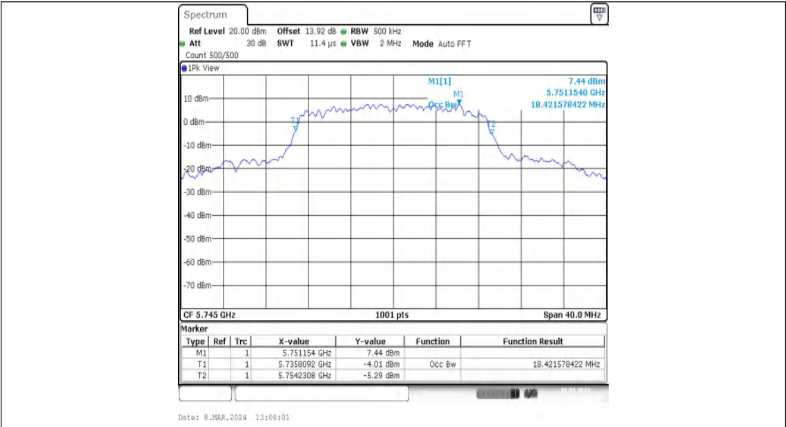
11N20MIMO-Ant1-5745
