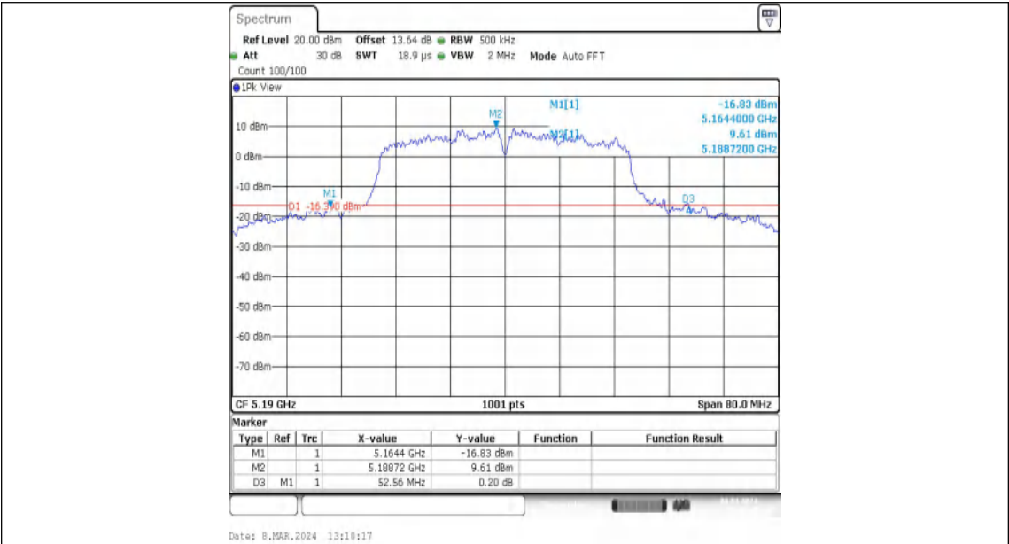
11N40MIMO-Ant1-5190
