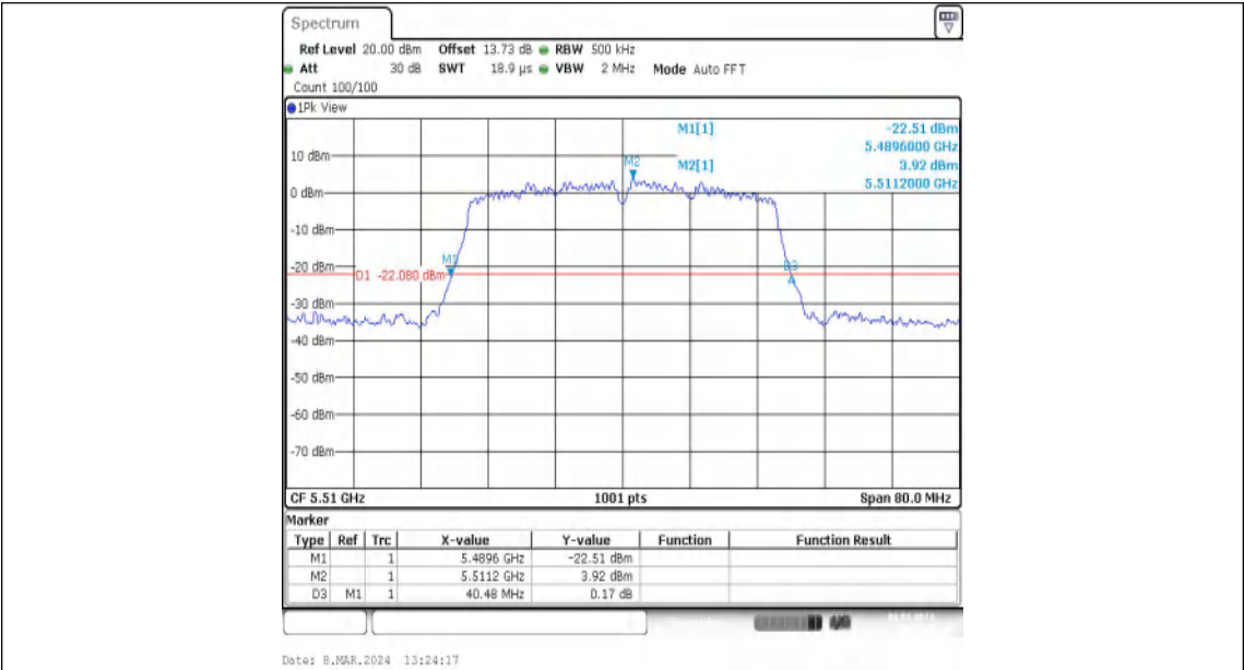
11N40MIMO-Ant1-5510
