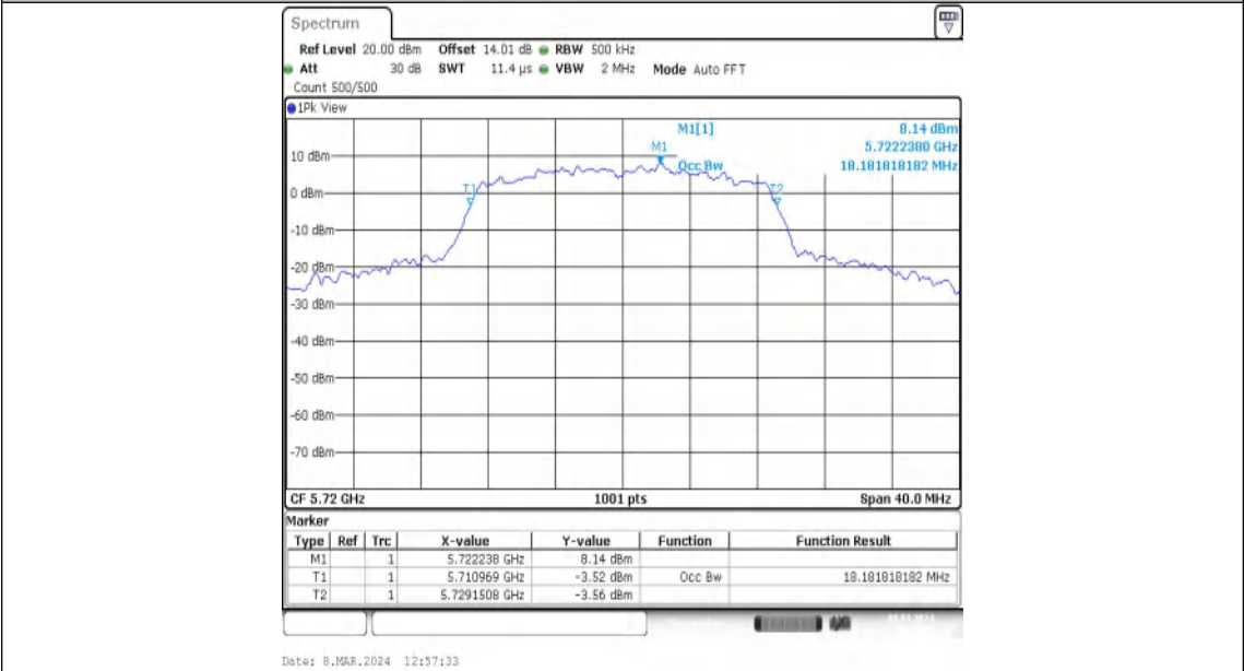
11N20MIMO-Ant2-5720
