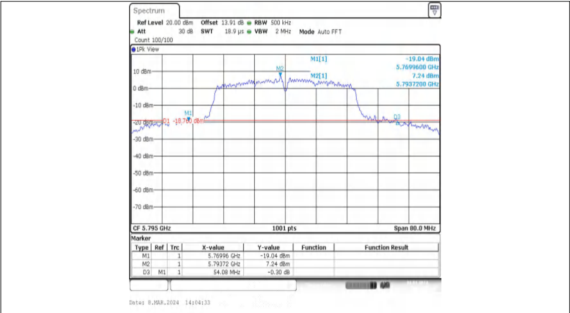
11N40MIMO-Ant1-5795
