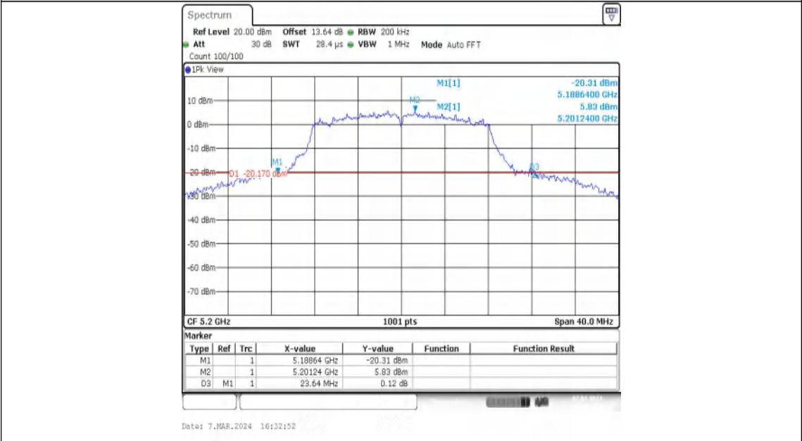
11A-Ant1-5200
