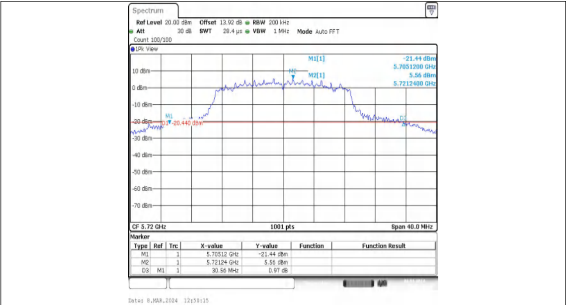
11N20MIMO-Ant1-5720
