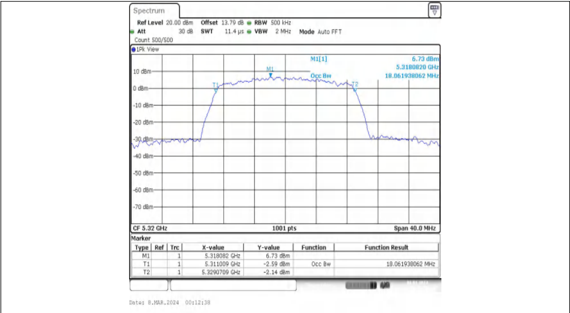
11N20MIMO-Ant1-5320
