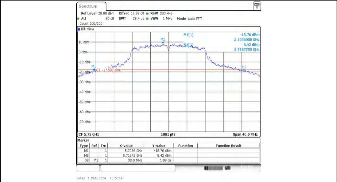
11A-Ant1-5720
