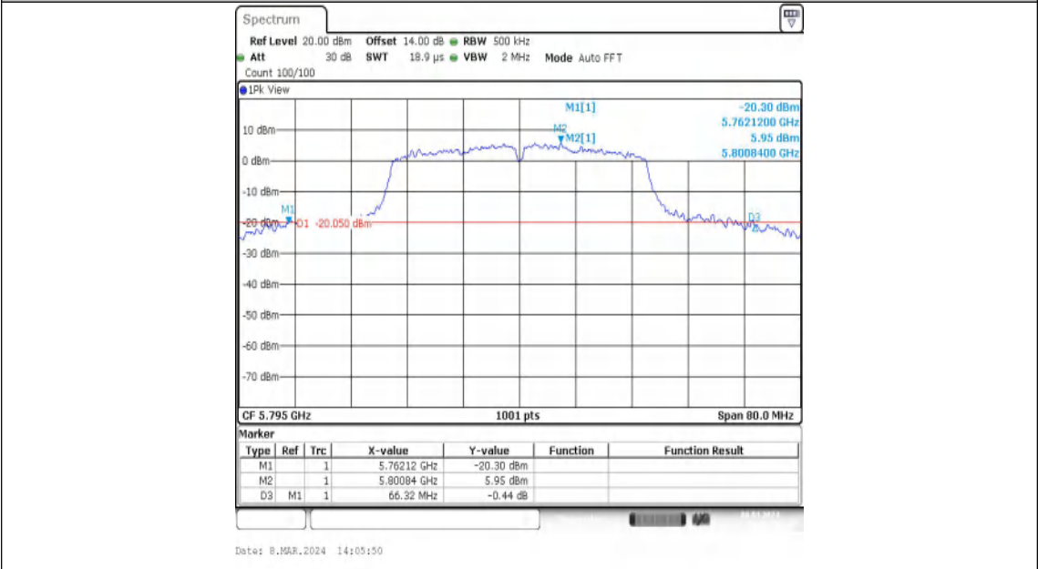
11N40MIMO-Ant2-5795
