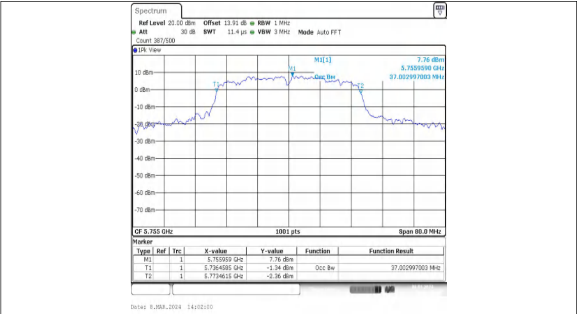
11N40MIMO-Ant1-5755
