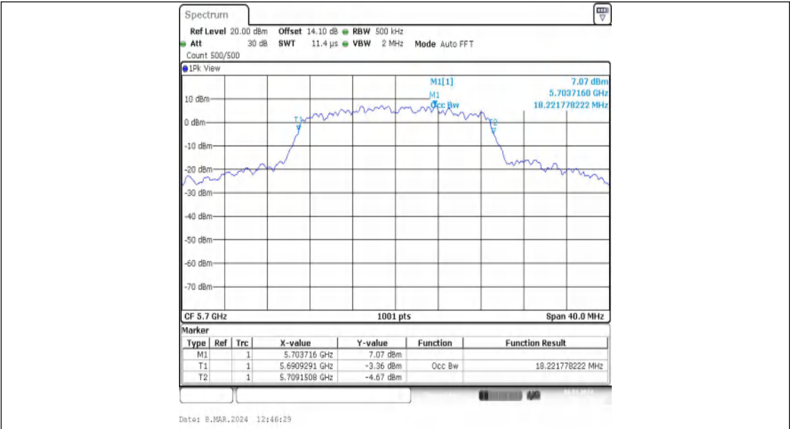
11N20MIMO-Ant1-5700
