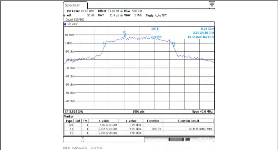
11N20MIMO-Ant1-5825
