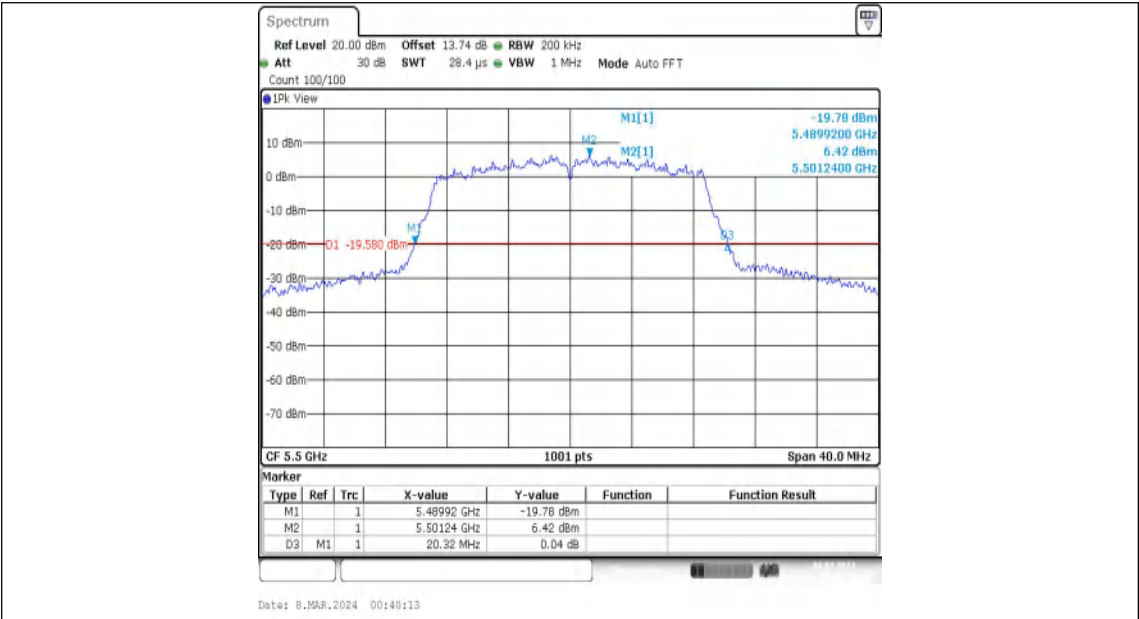
11N20MIMO-Ant1-5500
