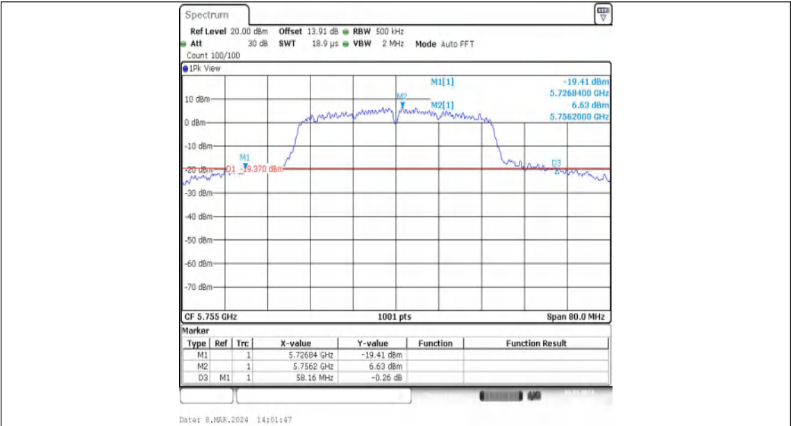
11N40MIMO-Ant1-5755
