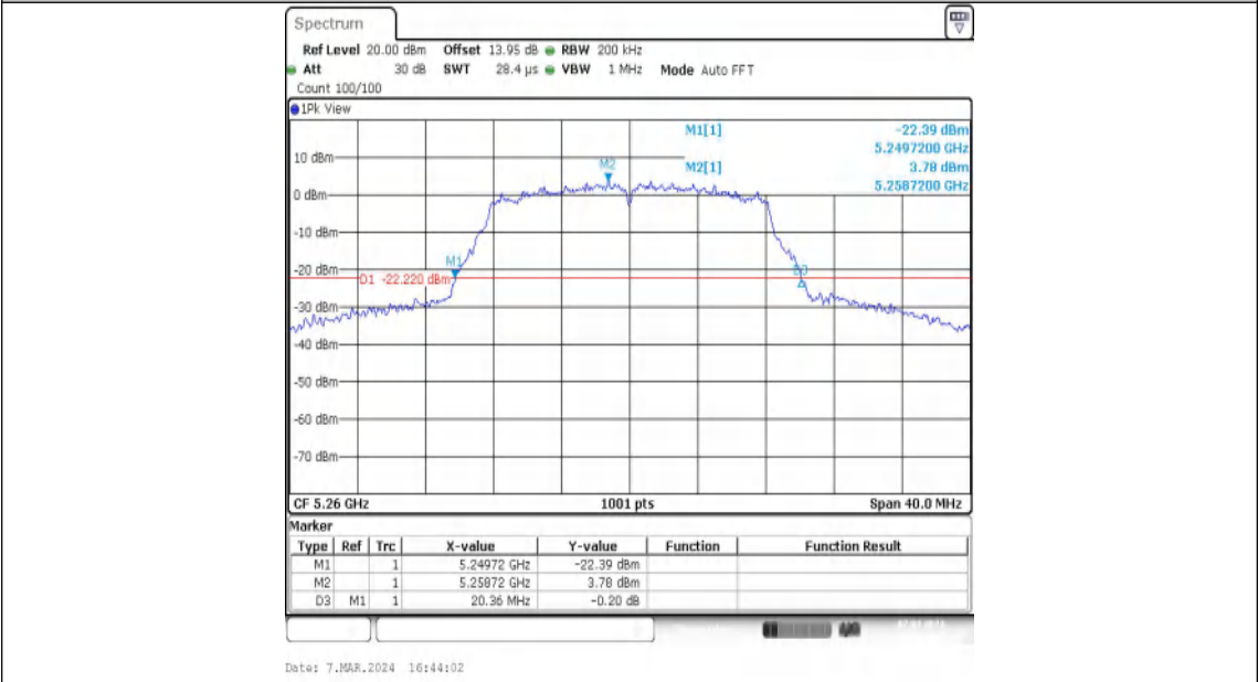
11A-Ant1-5260
