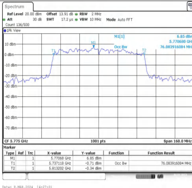
11AC80MIMO-Ant1-5775
