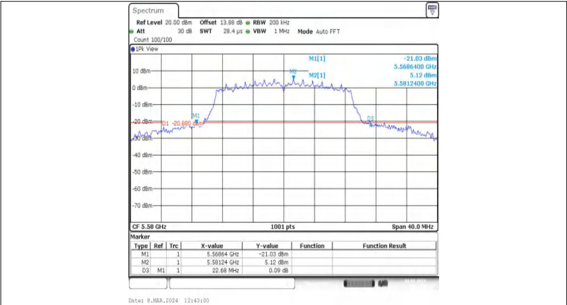
11N20MIMO-Ant1-5580
