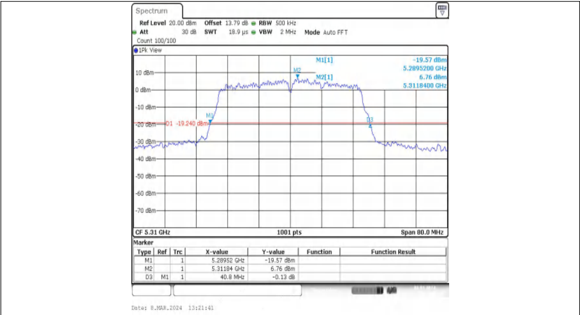
11N40MIMO-Ant1-5310
