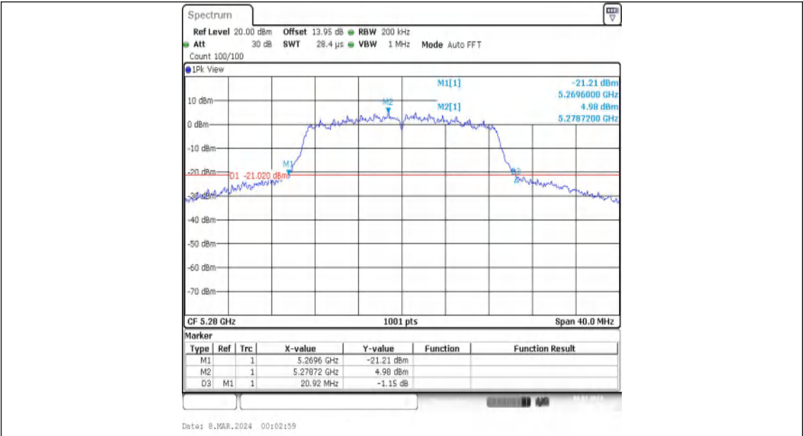
11N20MIMO-Ant1-5280
