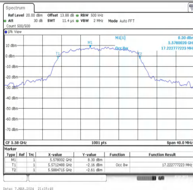
11A-Ant1-5580
