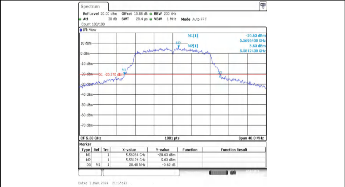
11A-Ant1-5580
