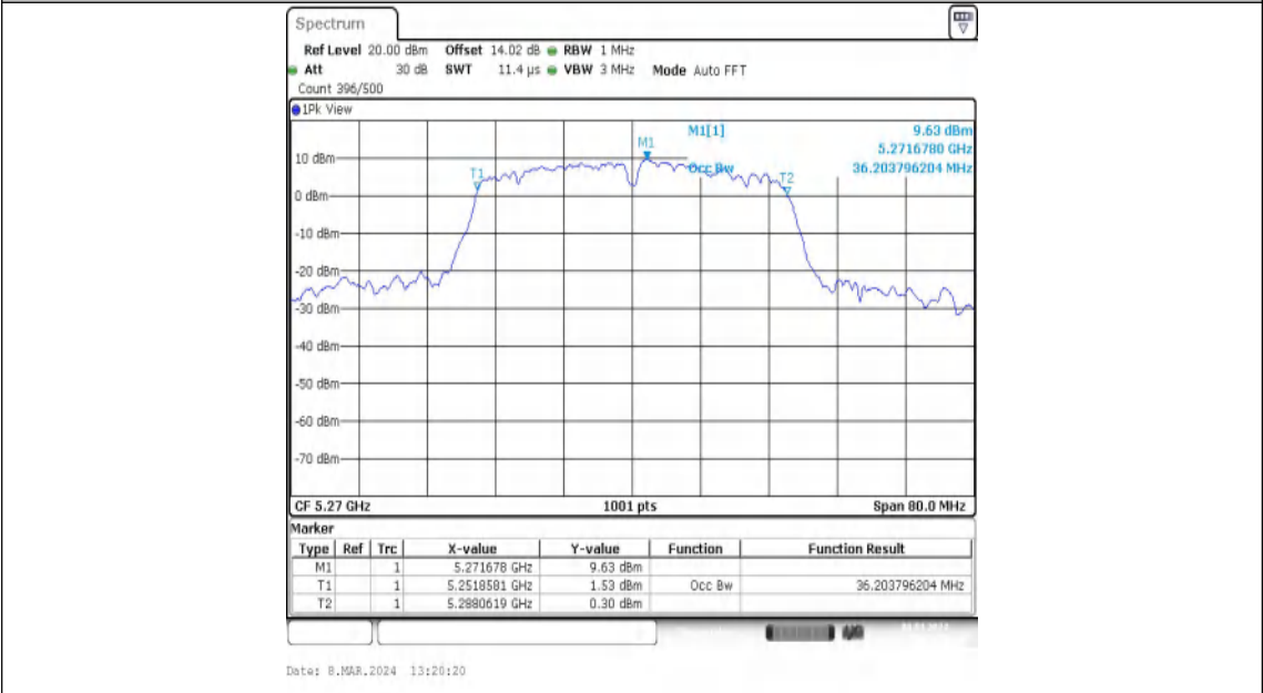
11N40MIMO-Ant2-5270
