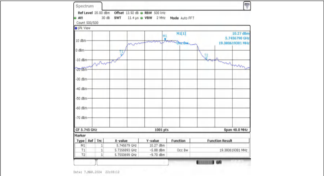
11A-Ant1-5745
