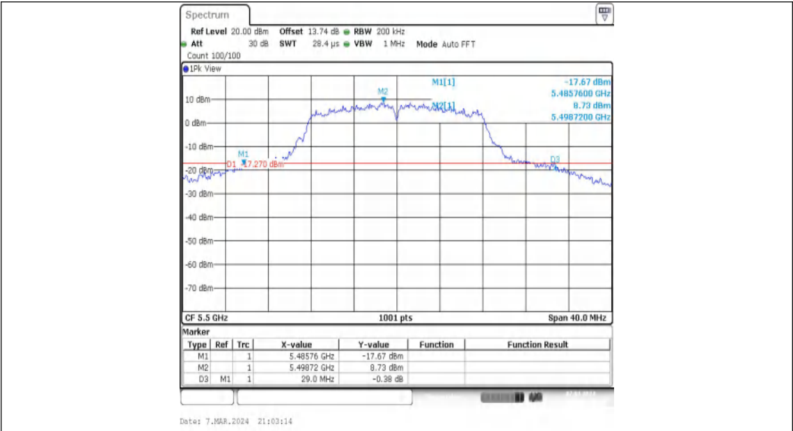
11A-Ant1-5500
