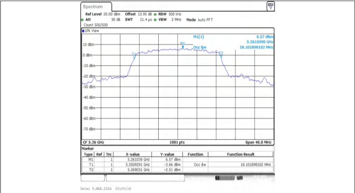
11N20MIMO-Ant1-5260
