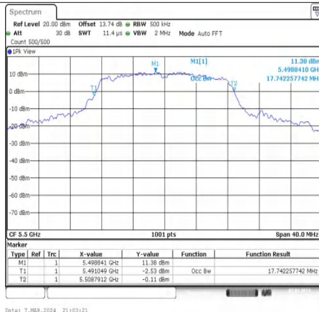
11A-Ant1-5500
