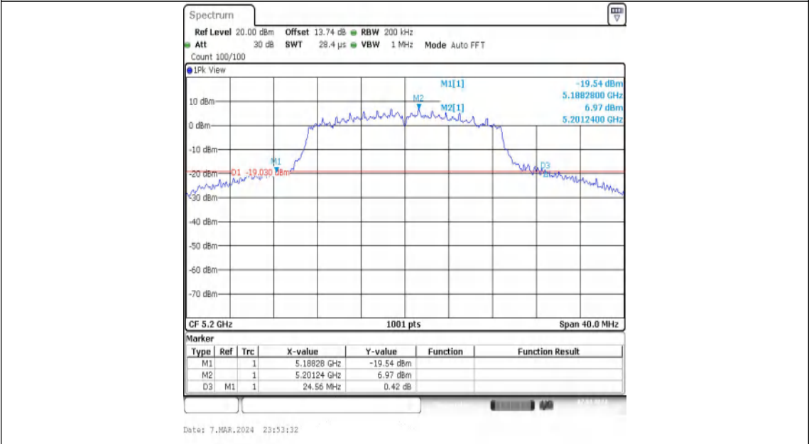
11N20MIMO-Ant2-5200
