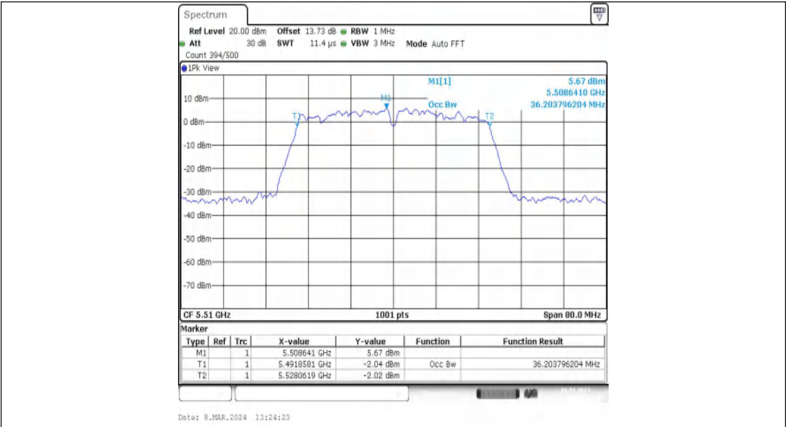
11N40MIMO-Ant1-5510
