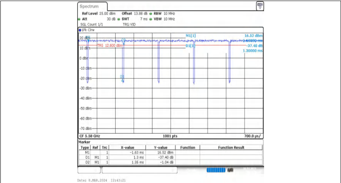
NTNV-11N20MIMO-Ant1-5580
