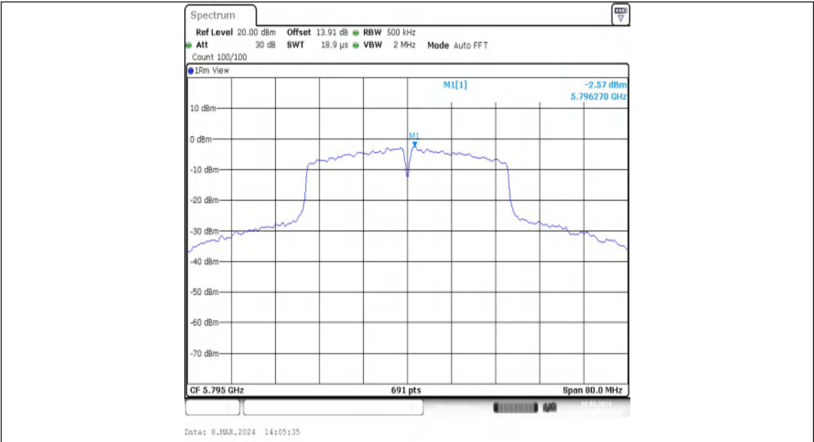
11N40MIMO-Ant1-5795-PASS
