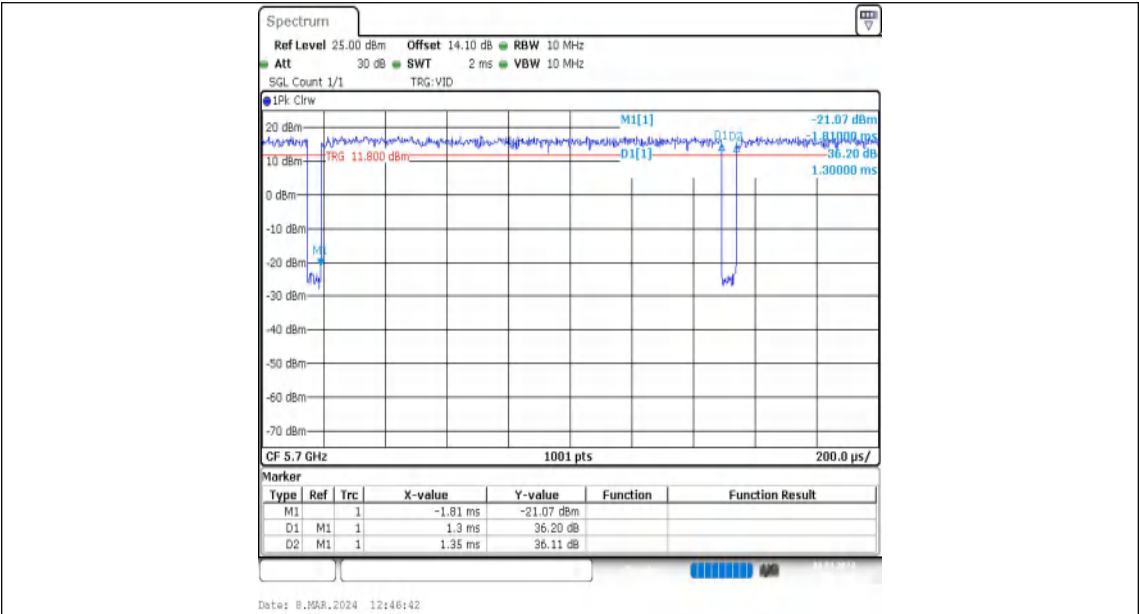
NTNV-11N20MIMO-Ant1-5700
