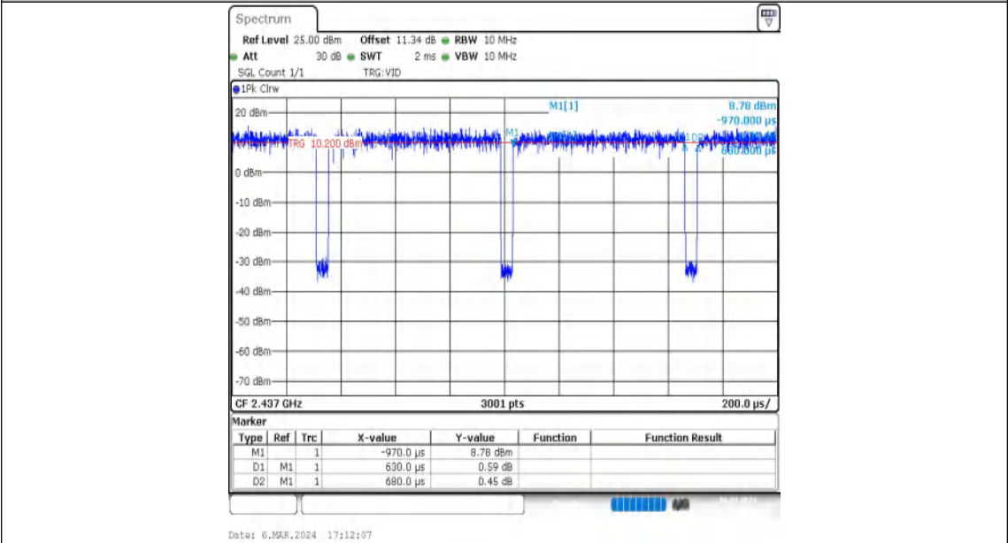
NTNV-11N40MIMO-Ant2-2437
