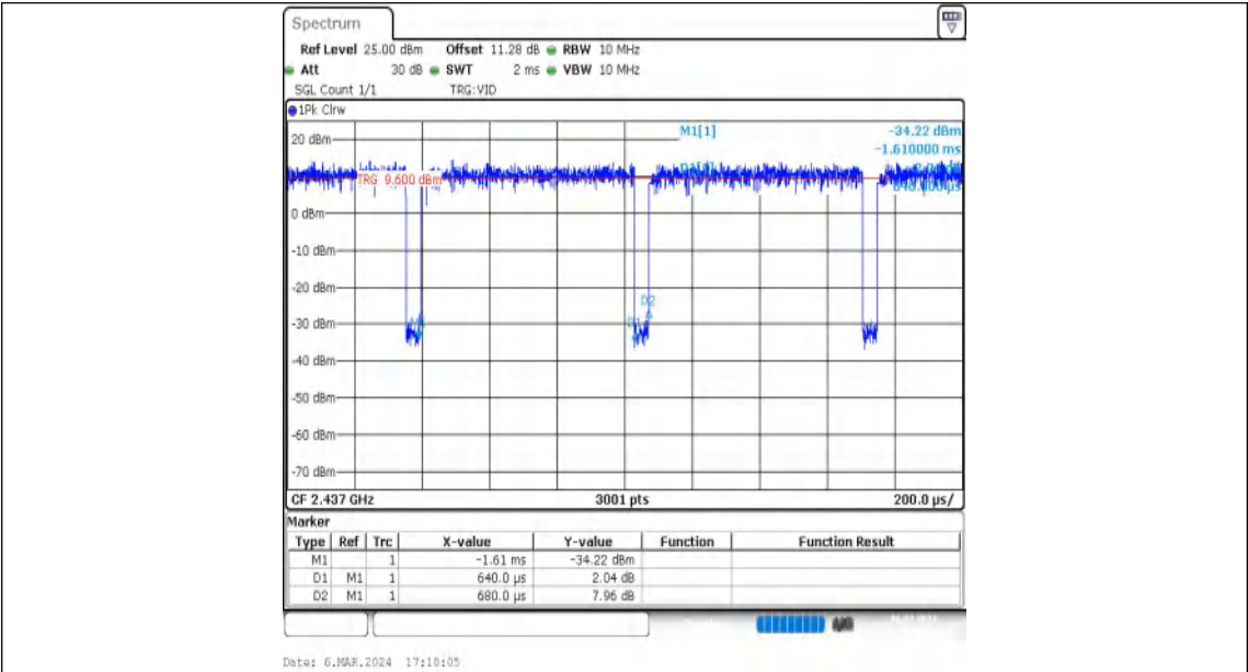
NTNV-11N40MIMO-Ant1-2437
