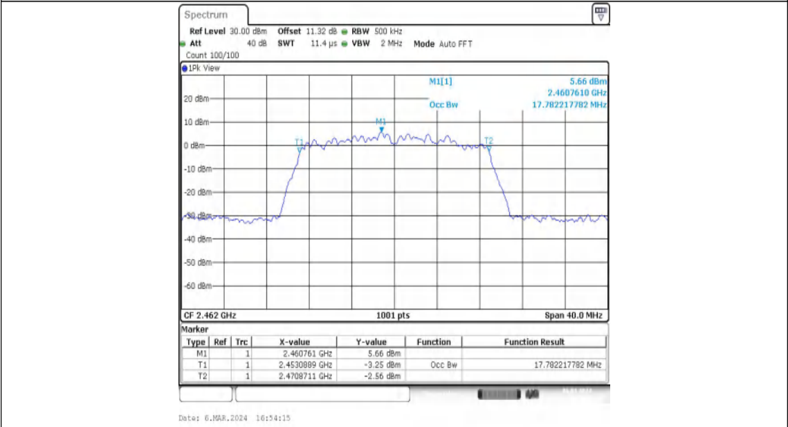
11N20MIMO-Ant1-2462
