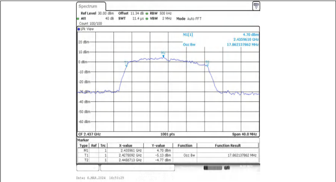
11N20MIMO-Ant2-2437
