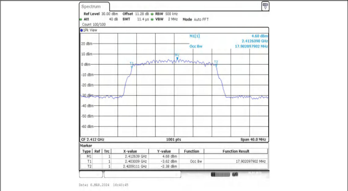
11N20MIMO-Ant1-2412
