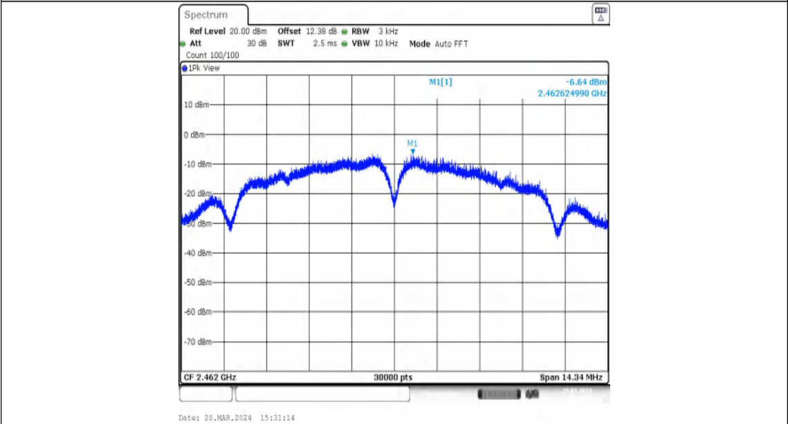
11B-Ant2-2462-PASS
