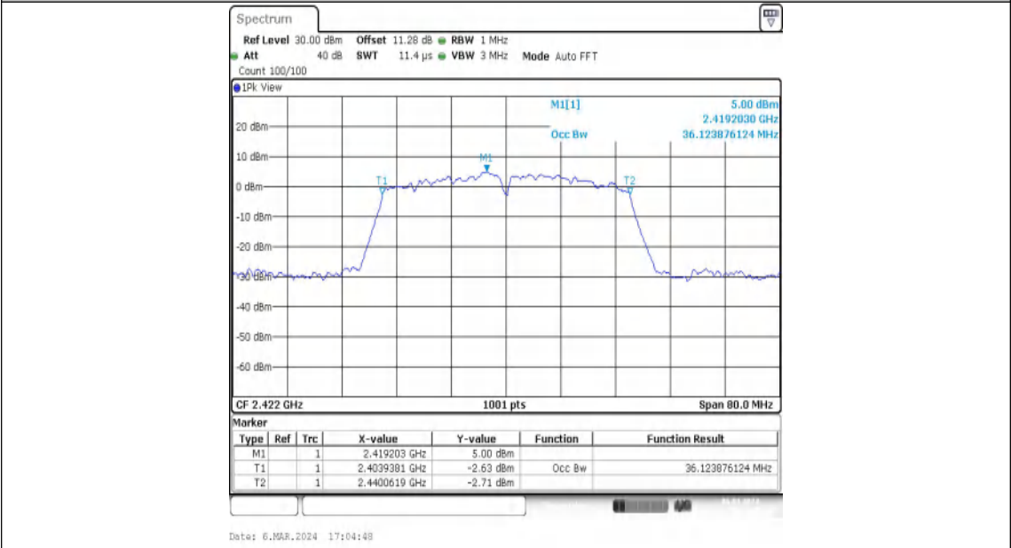
11N40MIMO-Ant1-2422
