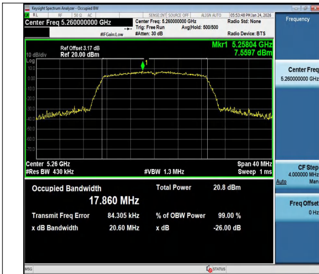
11ac20MIMO-Ant1-5260
