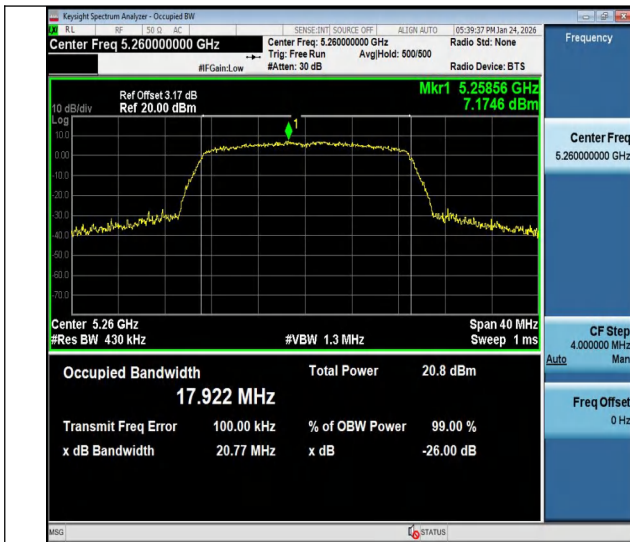
11n20MIMO-Ant1-5260
