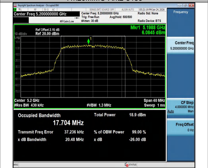
11n20MIMO-Ant2-5200
