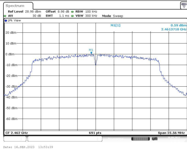
11N20SISO_Ant2_2462
