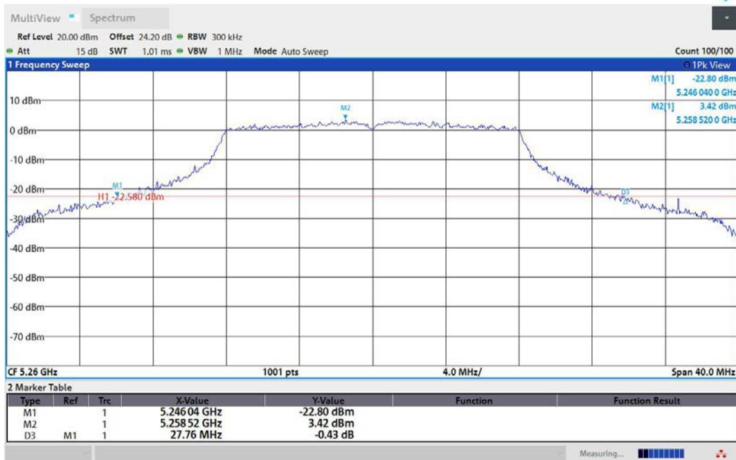
11A-Ant1-5260
