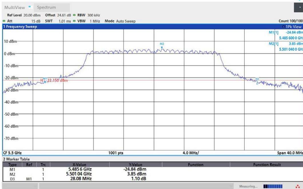
11N20MIMO-Ant2-5500
