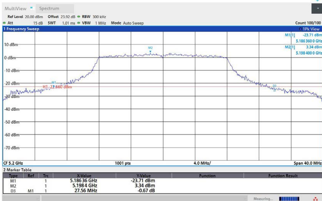
11A-Ant1-5200
