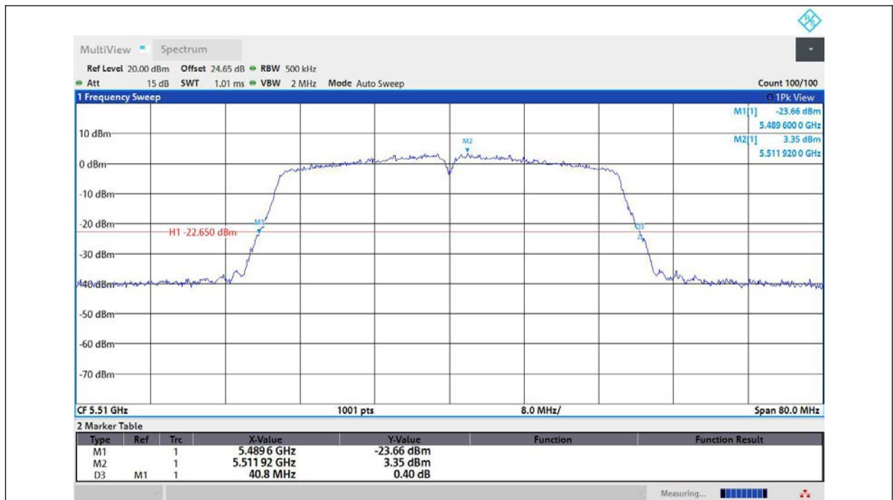
11N40MIMO-Ant1-5510
