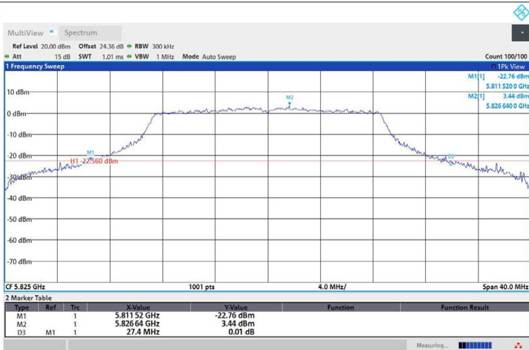
11N20MIMO-Ant1-5825
