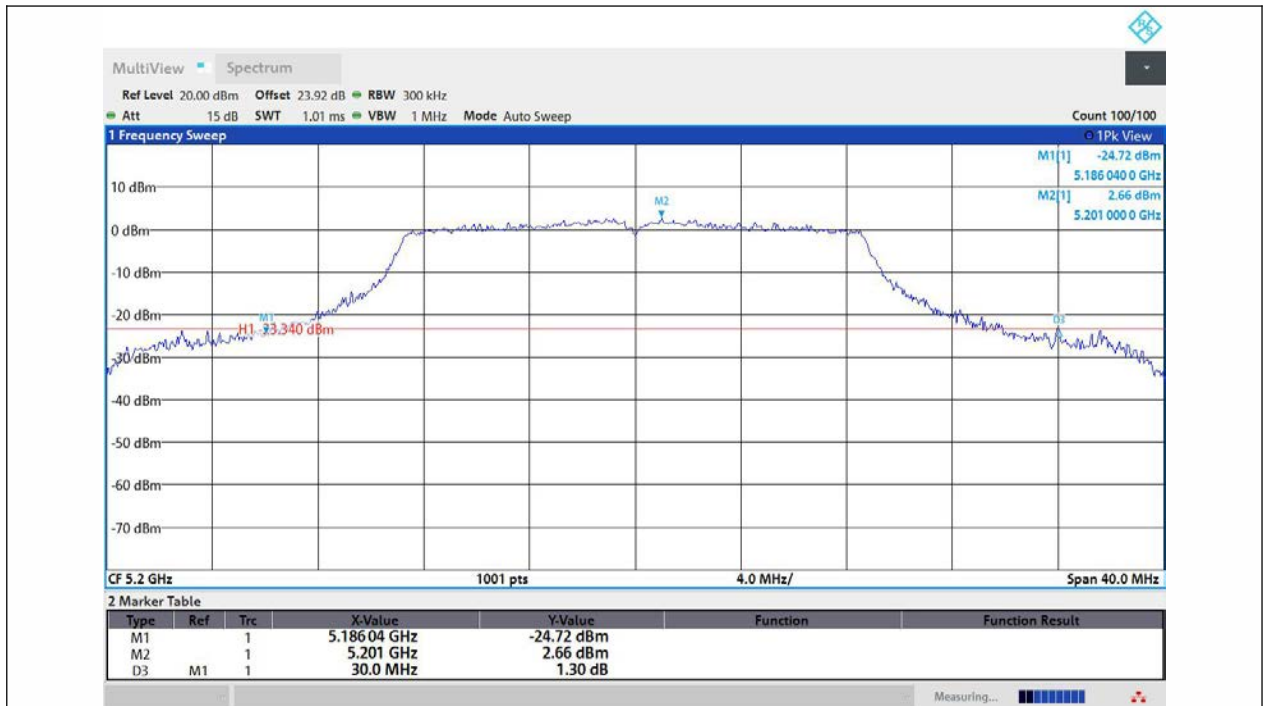
11AC20MIMO-Ant1-5200
