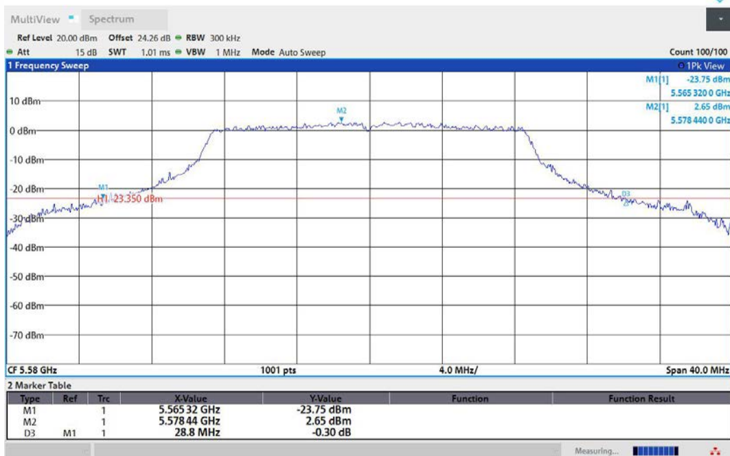
11N20MIMO-Ant1-5580
