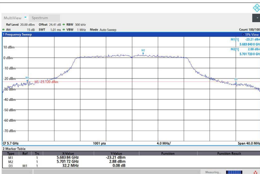
11N20MIMO-Ant1-5700
