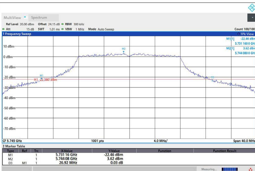
11A-Ant1-5745
