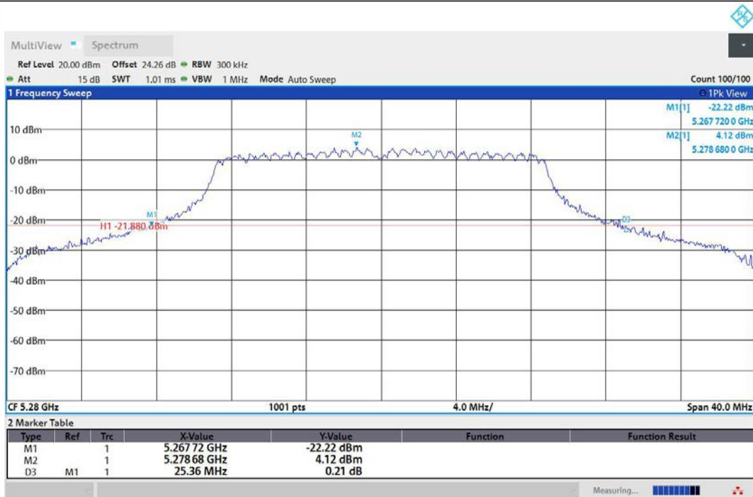
11N20MIMO-Ant2-5280
