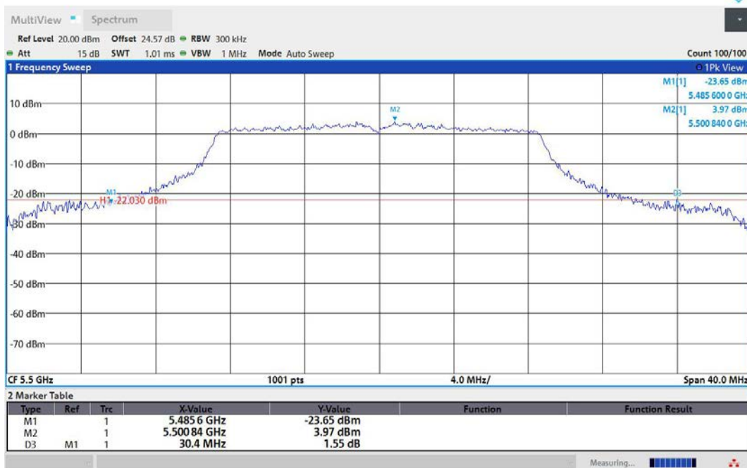
11N20MIMO-Ant1-5500
