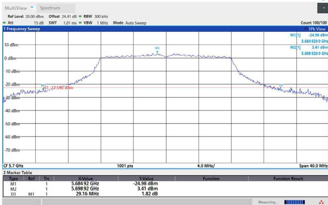
11A-Ant1-5700
