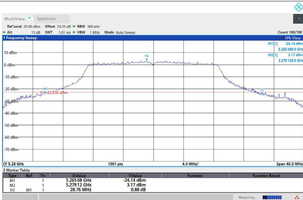
11N20MIMO-Ant1-5280
