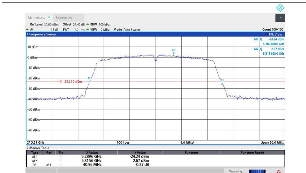
11N40MIMO-Ant1-5310
