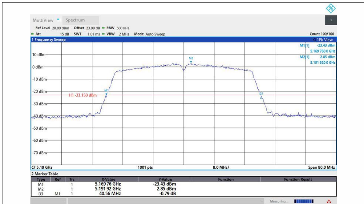
11N40MIMO-Ant1-5190
