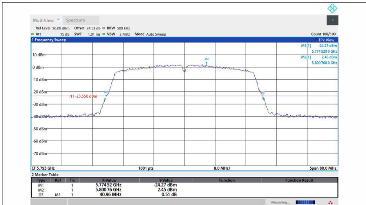
11N40MIMO-Ant1-5795
