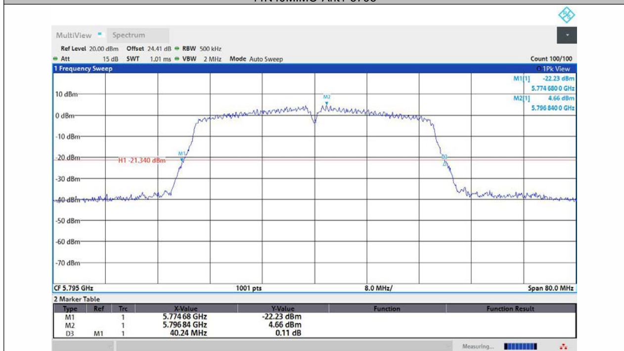
11N40MIMO-Ant2-5795
