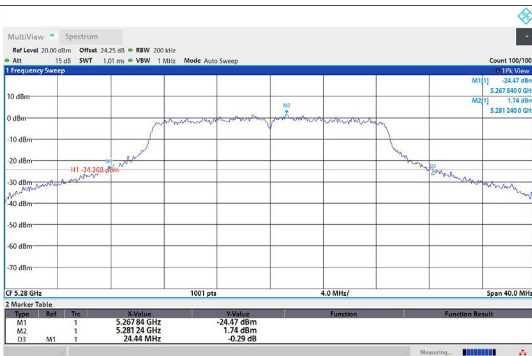
11AC20MIMO-Ant1-5280
