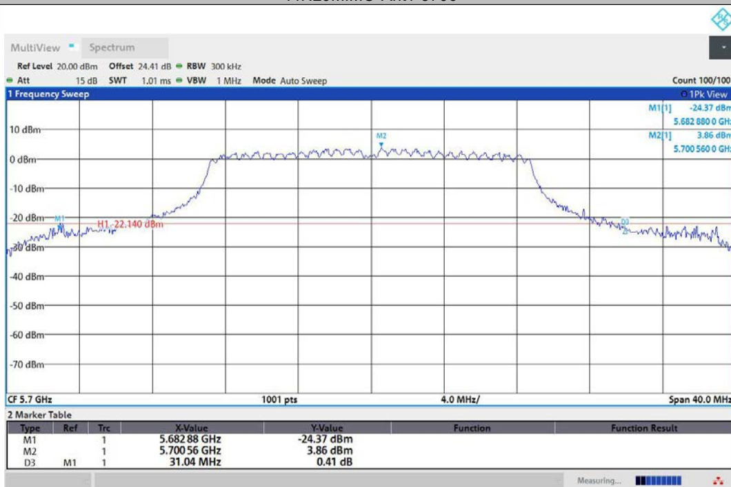
11N20MIMO-Ant2-5700
