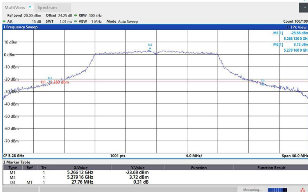
11A-Ant1-5280
