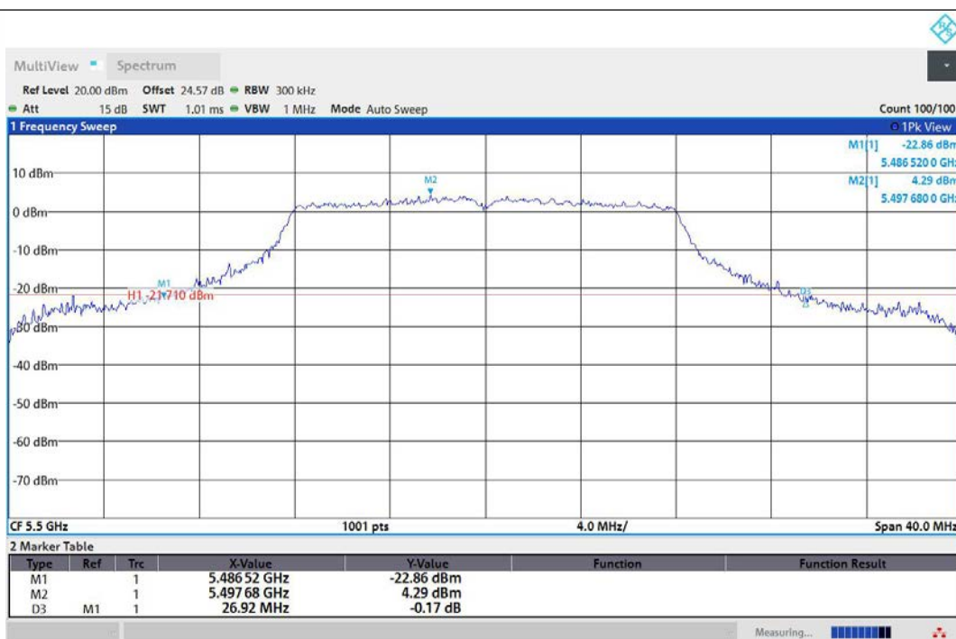
11A-Ant1-5500
