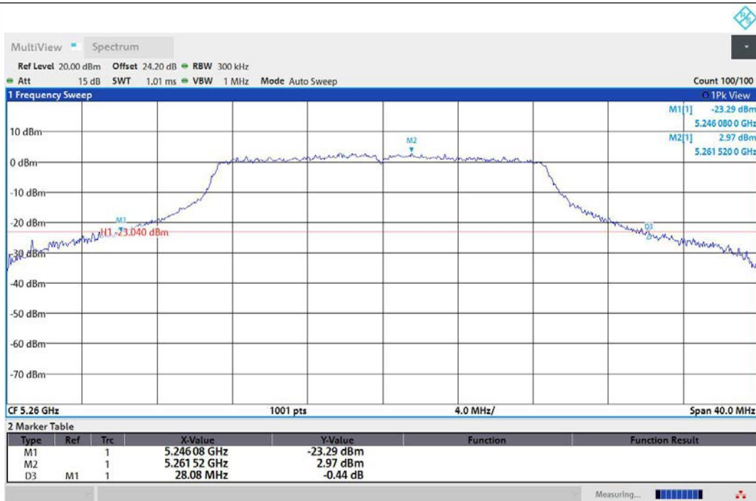
11N20MIMO-Ant1-5260
