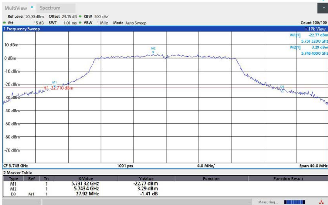
11N20MIMO-Ant1-5745
