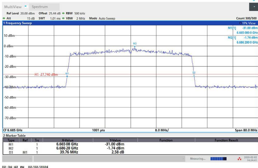
11AX40MIMO-Ant1-6685
