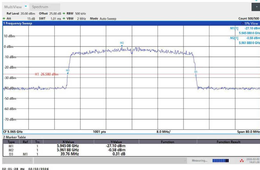
11AX40MIMO-Ant1-5965
