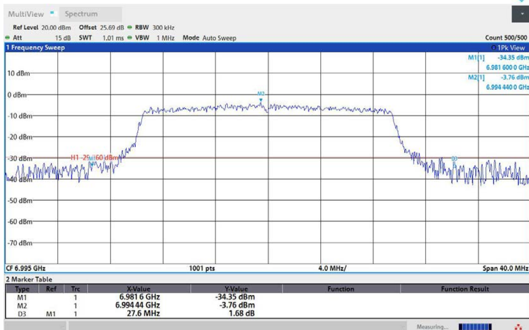
11AX20MIMO-Ant2-6995
