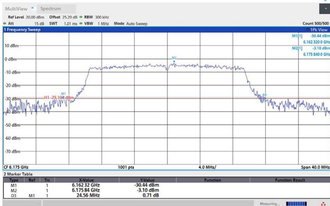
11AX20MIMO-Ant1-6175
