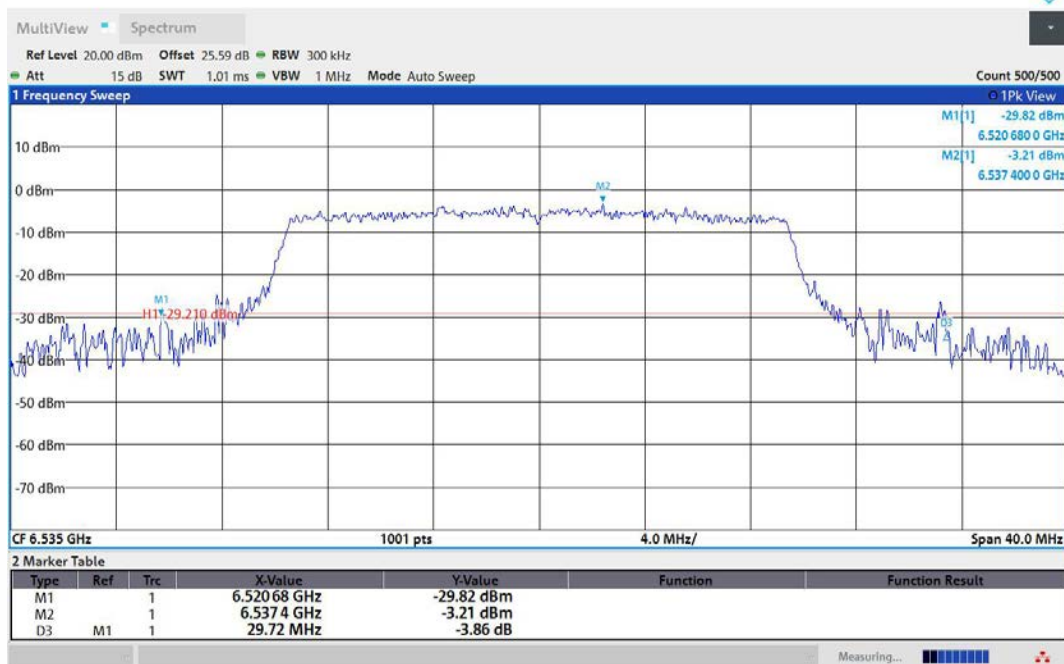
11AX20MIMO-Ant1-6535
