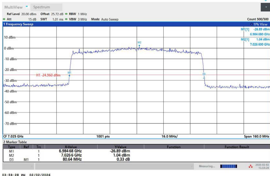
11AX80MIMO-Ant1-7025
