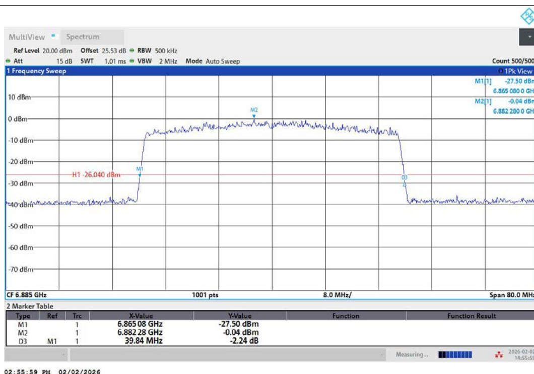
11AX40MIMO-Ant1-6885
