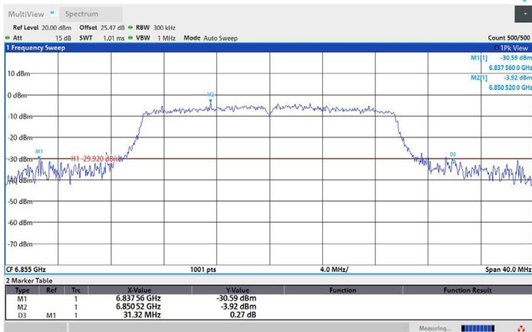
11AX20MIMO-Ant1-6855
