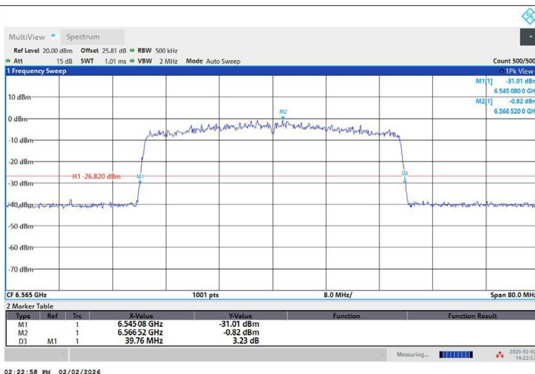
11AX40MIMO-Ant1-6565
