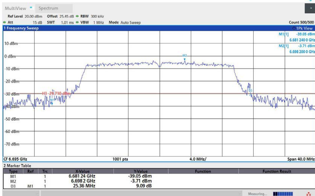
11AX20MIMO-Ant1-6695
