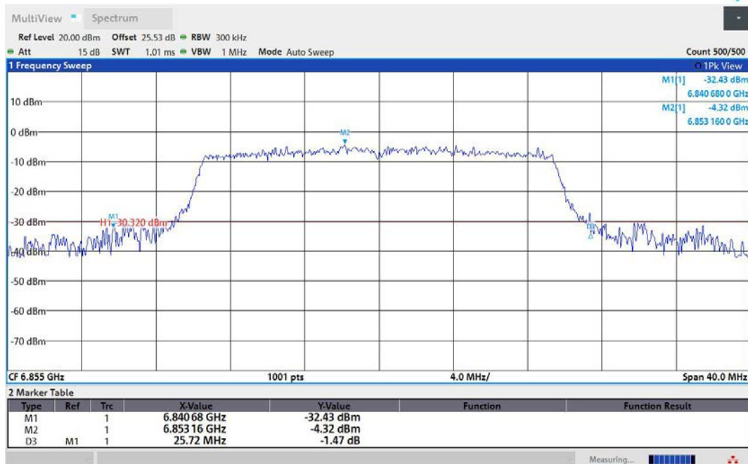
11AX20MIMO-Ant2-6855
