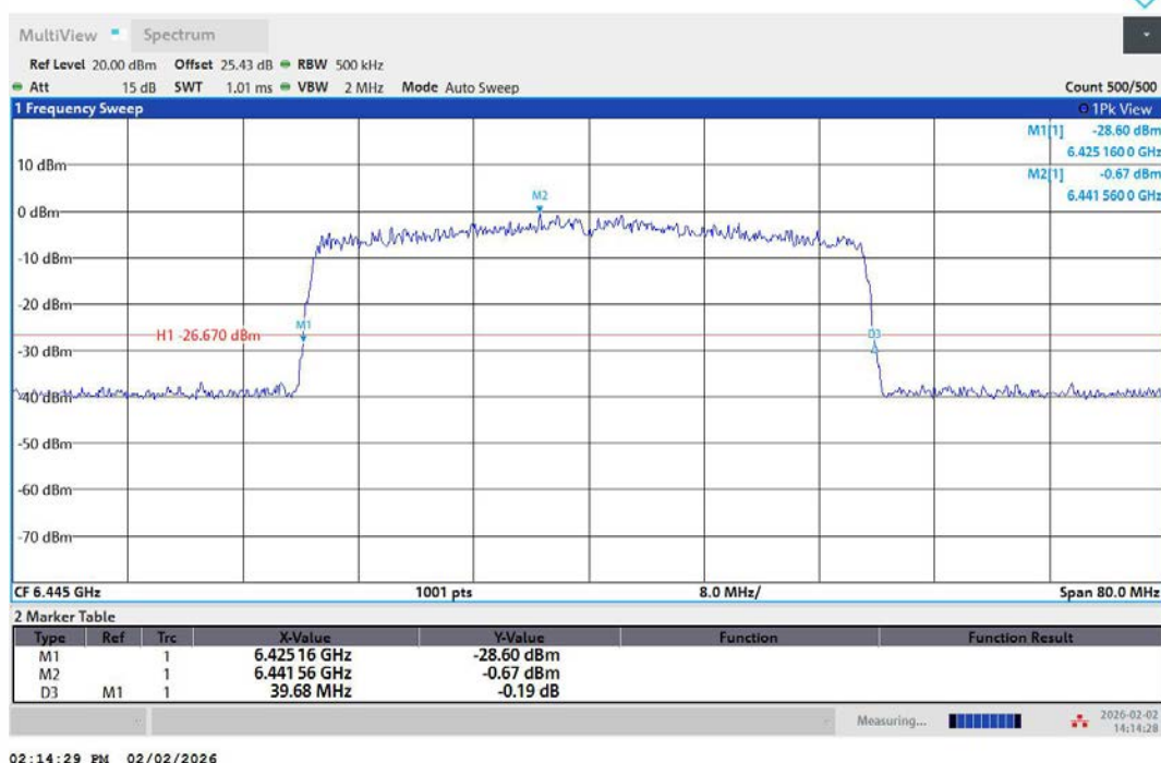
11AX40MIMO-Ant2-6445
