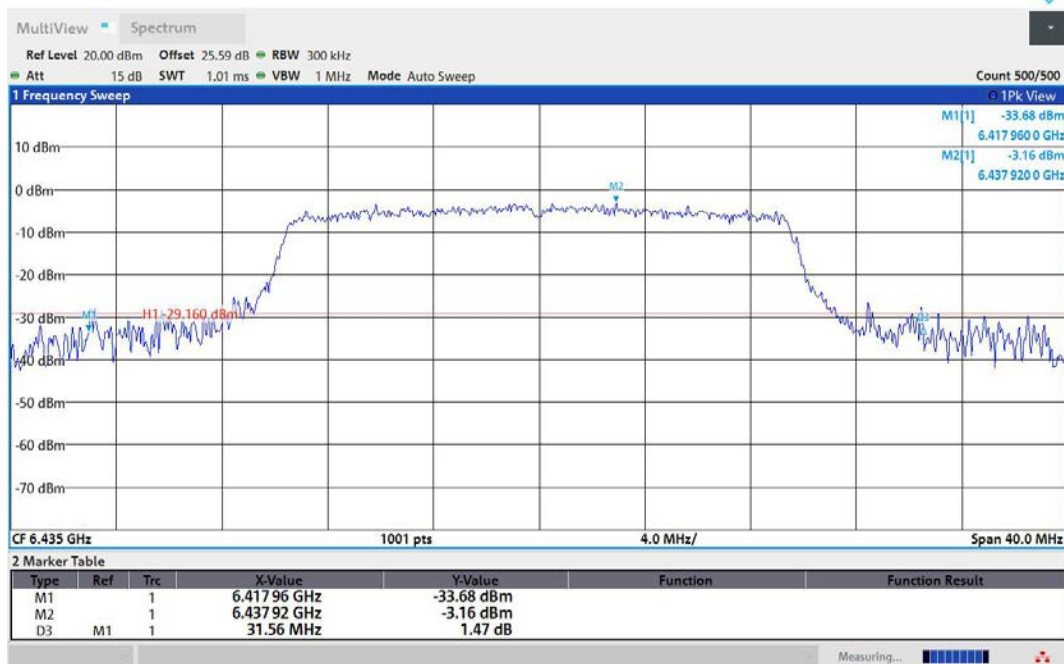
11AX20MIMO-Ant1-6435
