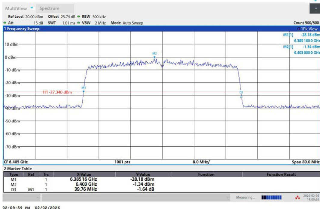
11AX40MIMO-Ant1-6405
