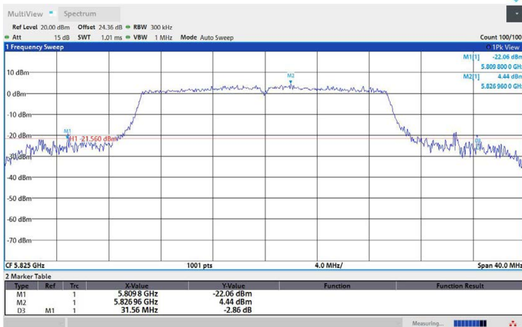
11AX20MIMO-Ant1-5825
