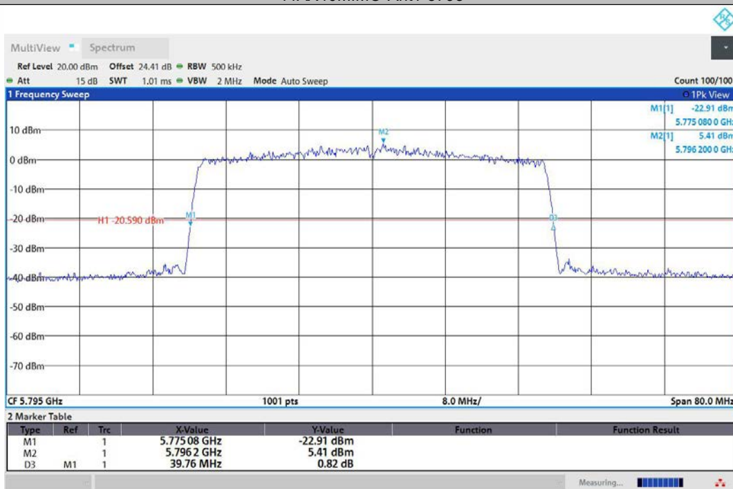
11AX40MIMO-Ant2-5795
