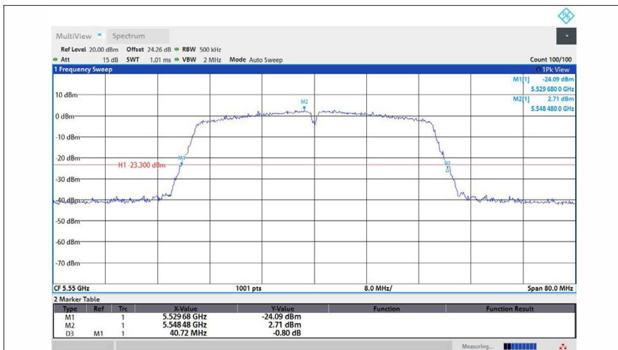
11AC40MIMO-Ant1-5550
