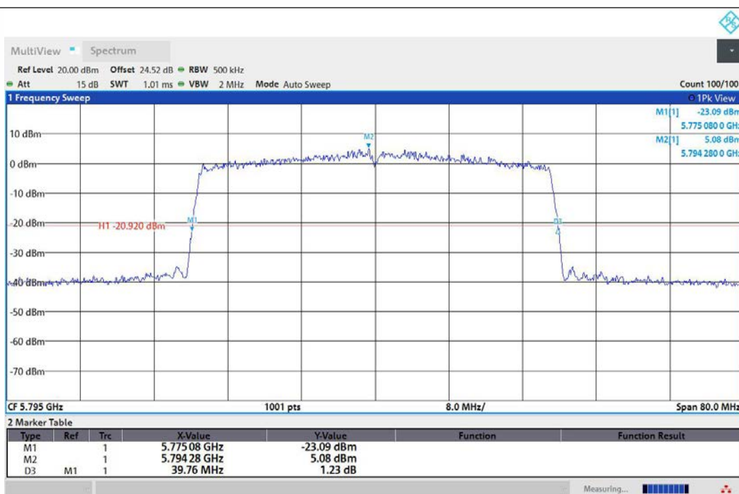
11AX40MIMO-Ant1-5795
