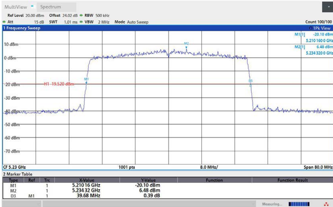
11AX40MIMO-Ant2-5230
