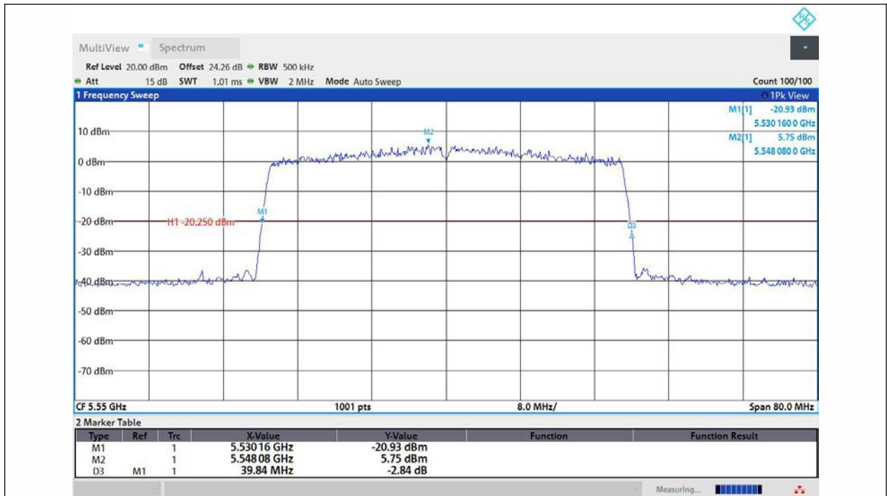
11AX40MIMO-Ant1-5550
