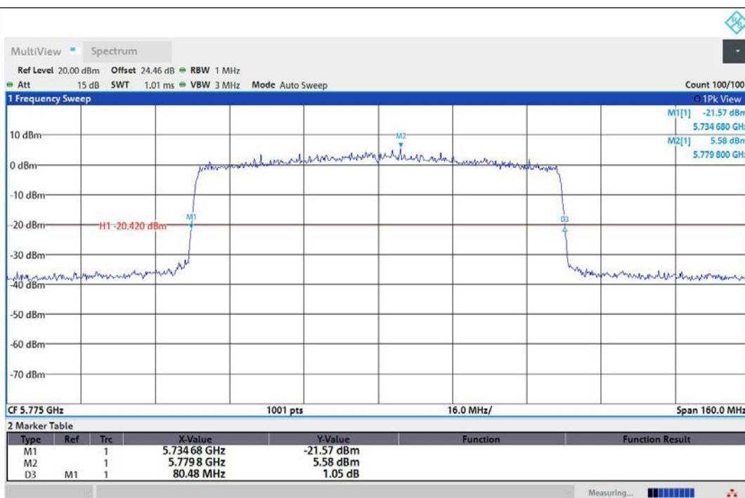
11AX80MIMO-Ant1-5775
