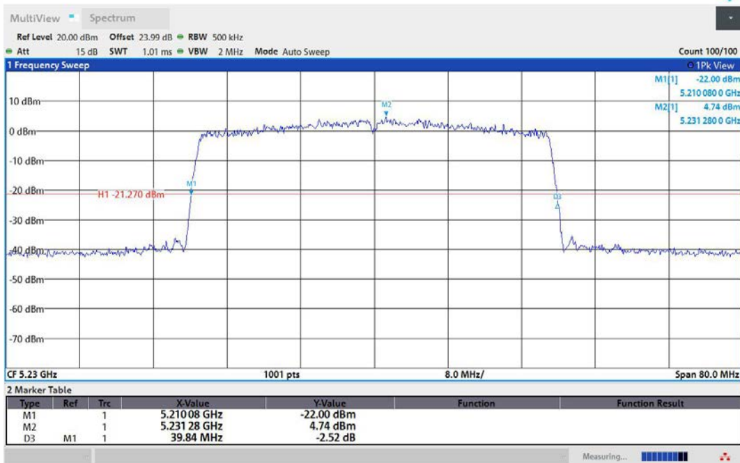
11AX40MIMO-Ant1-5230
