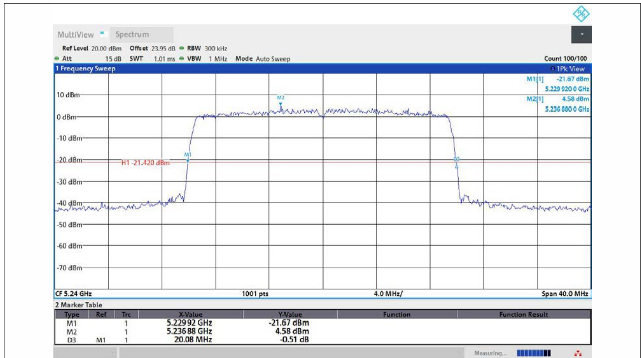
11AX20MIMO-Ant1-5240
