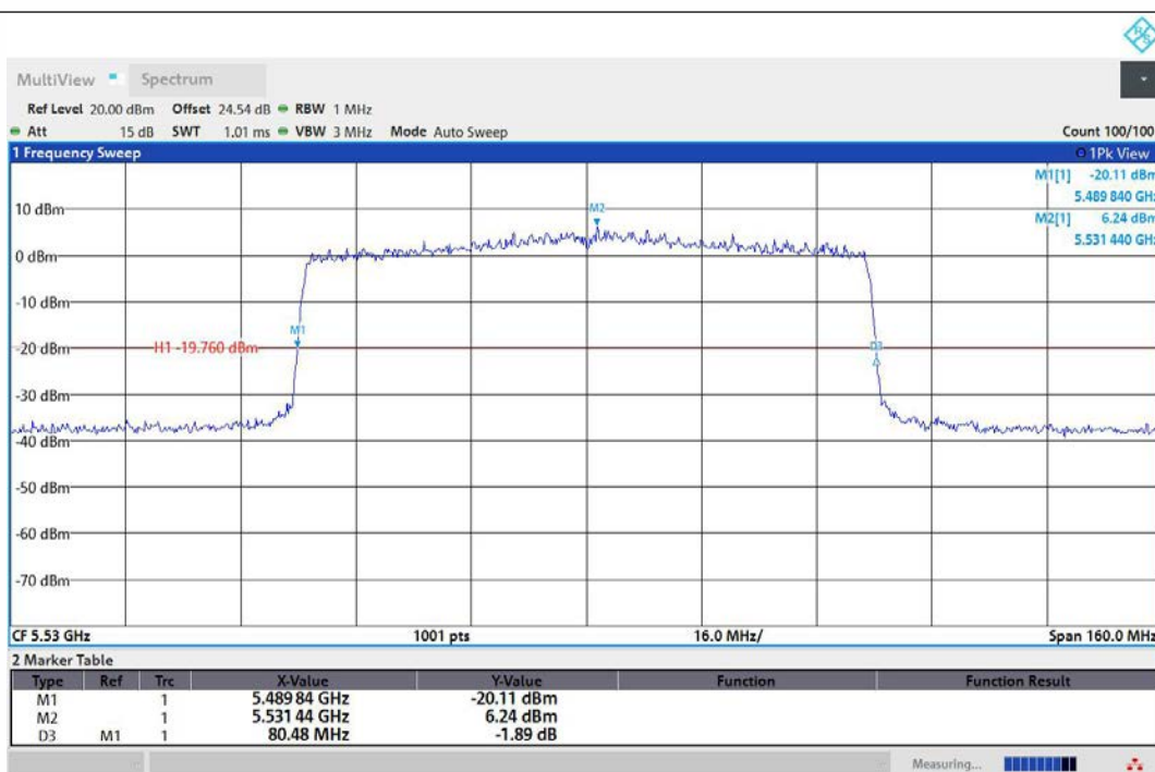
11AX80MIMO-Ant1-5530
