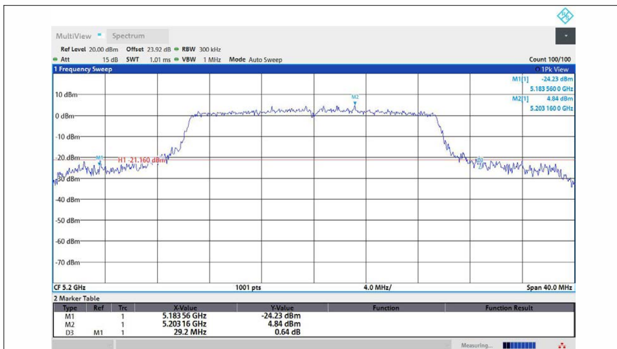
11AX20MIMO-Ant1-5200
