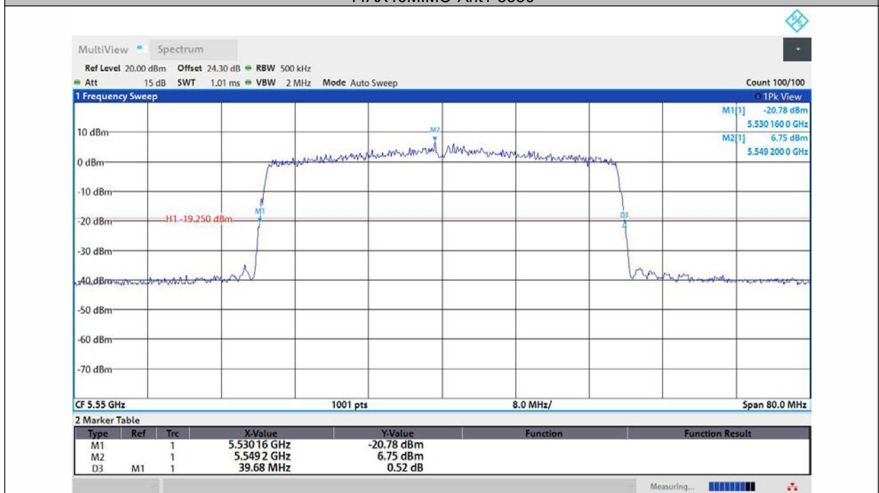
11AX40MIMO-Ant2-5550
