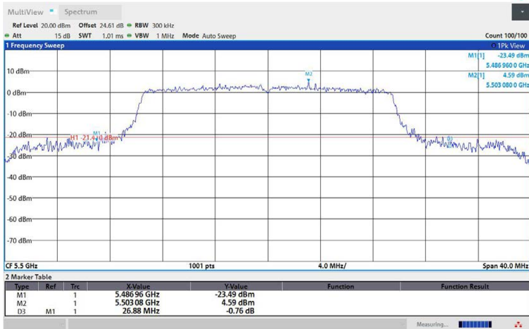
11AX20MIMO-Ant2-5500
