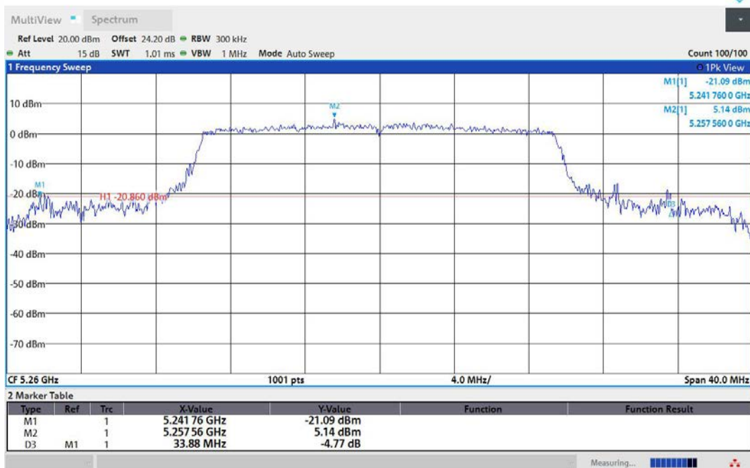
11AX20MIMO-Ant1-5260
