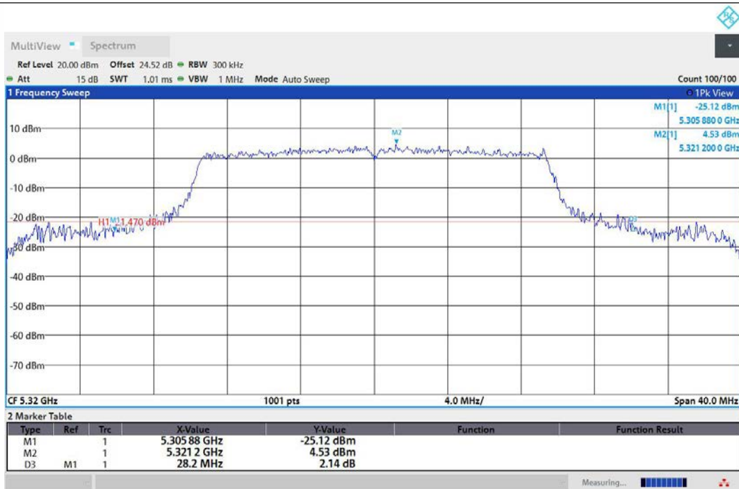
11AX20MIMO-Ant1-5320
