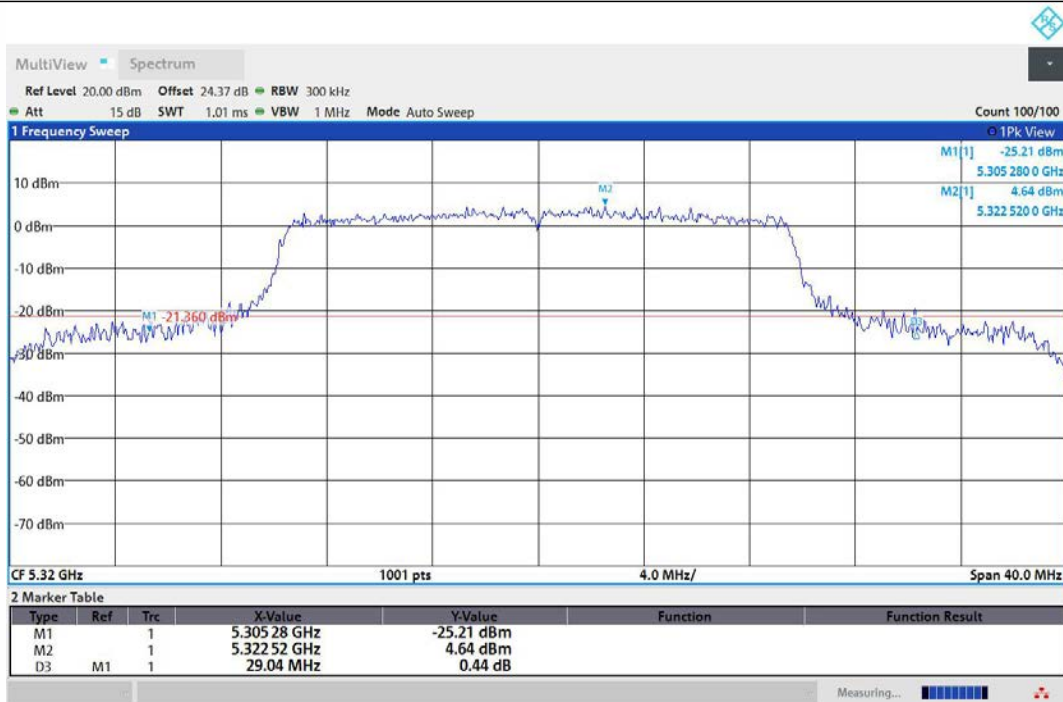
11AX20MIMO-Ant2-5320
