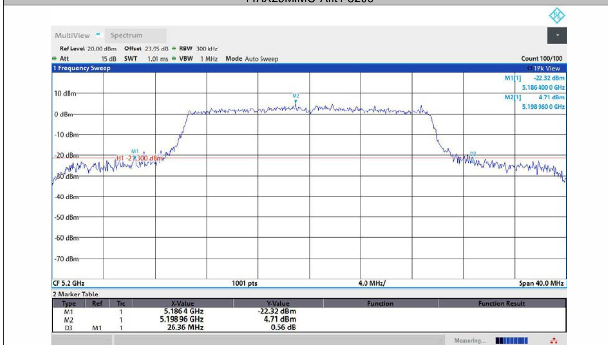
11AX20MIMO-Ant2-5200
